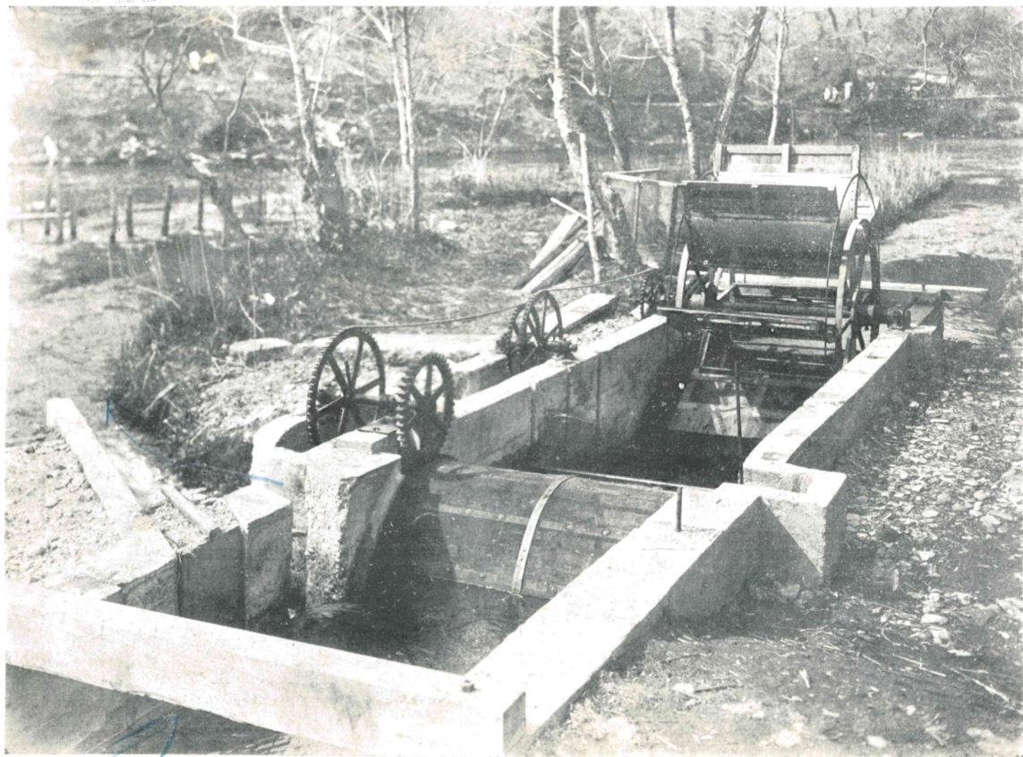
種魚流入防止装置
