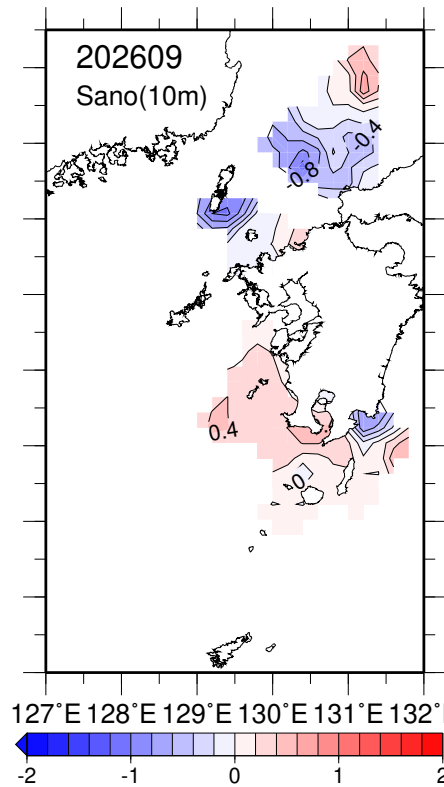
塩分平年偏差(10m深).
