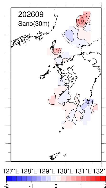
塩分平年偏差(30m深).
