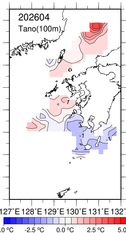
水温平年偏差(100m深).
