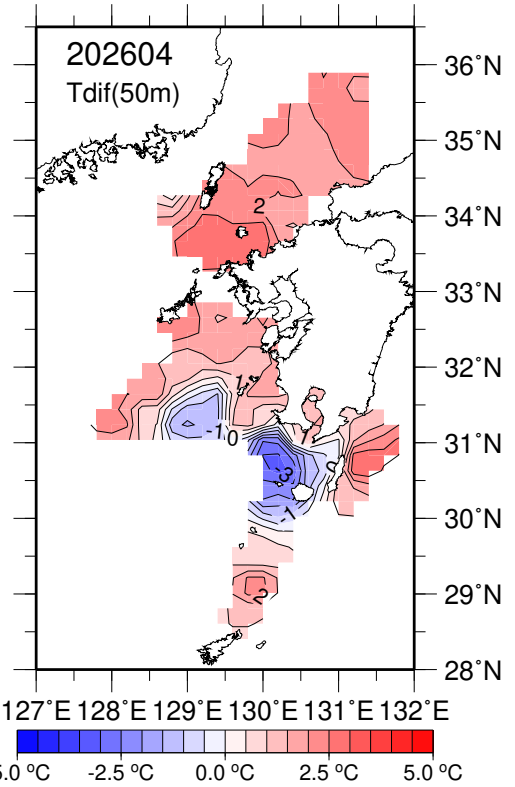
水温前年差(50m深).
