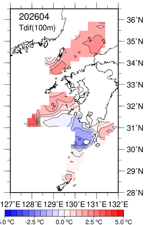
水温前年差(100m深).
