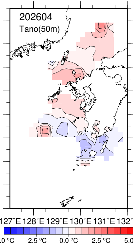
水温平年偏差(50m深).
