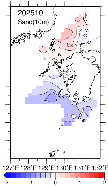
塩分平年偏差(10m深).
