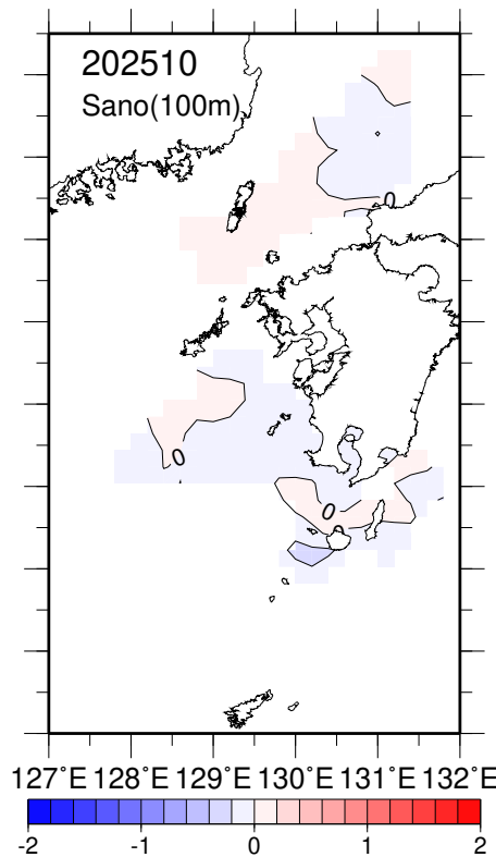
塩分平年偏差(100m深).
