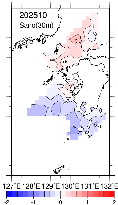
塩分平年偏差(30m深).
