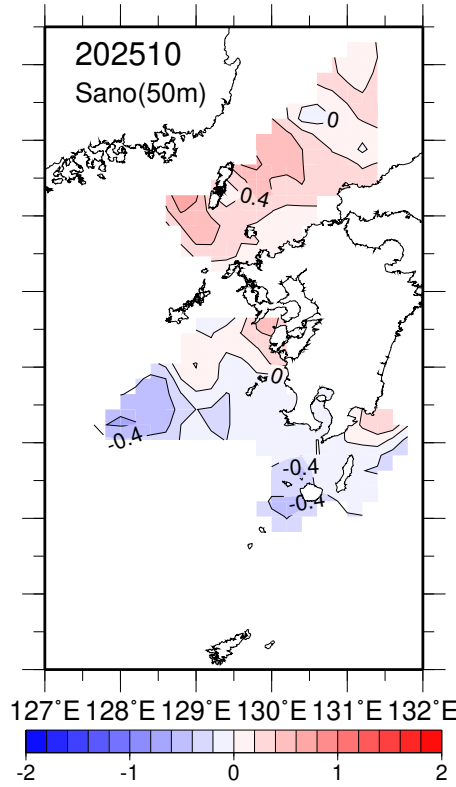
塩分平年偏差(50m深).
