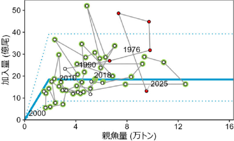
図7 再生産関係
