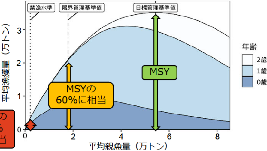
図8 管理基準値
