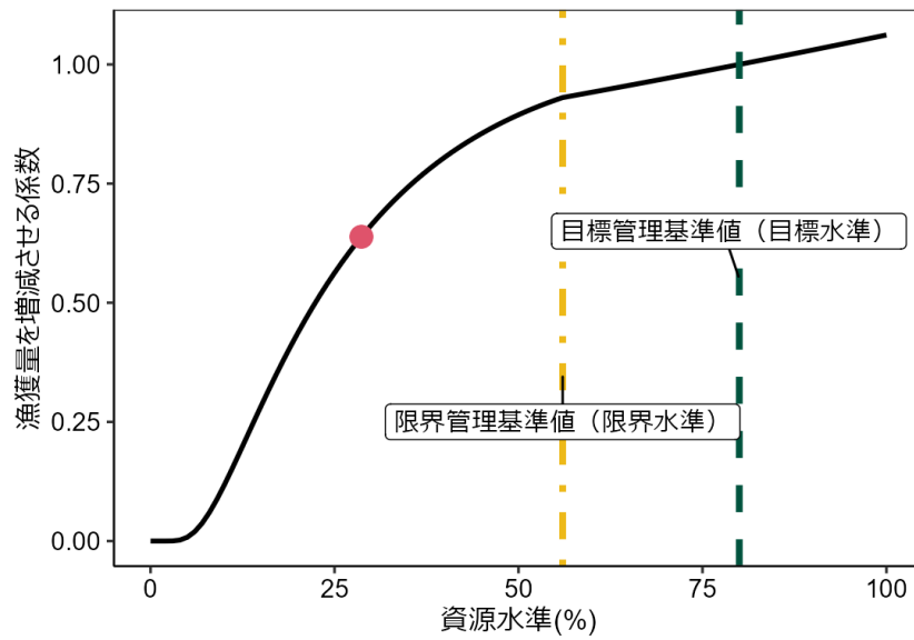
補足図 4-1. 変動緩和措置をとった場合の漁獲管理規則
