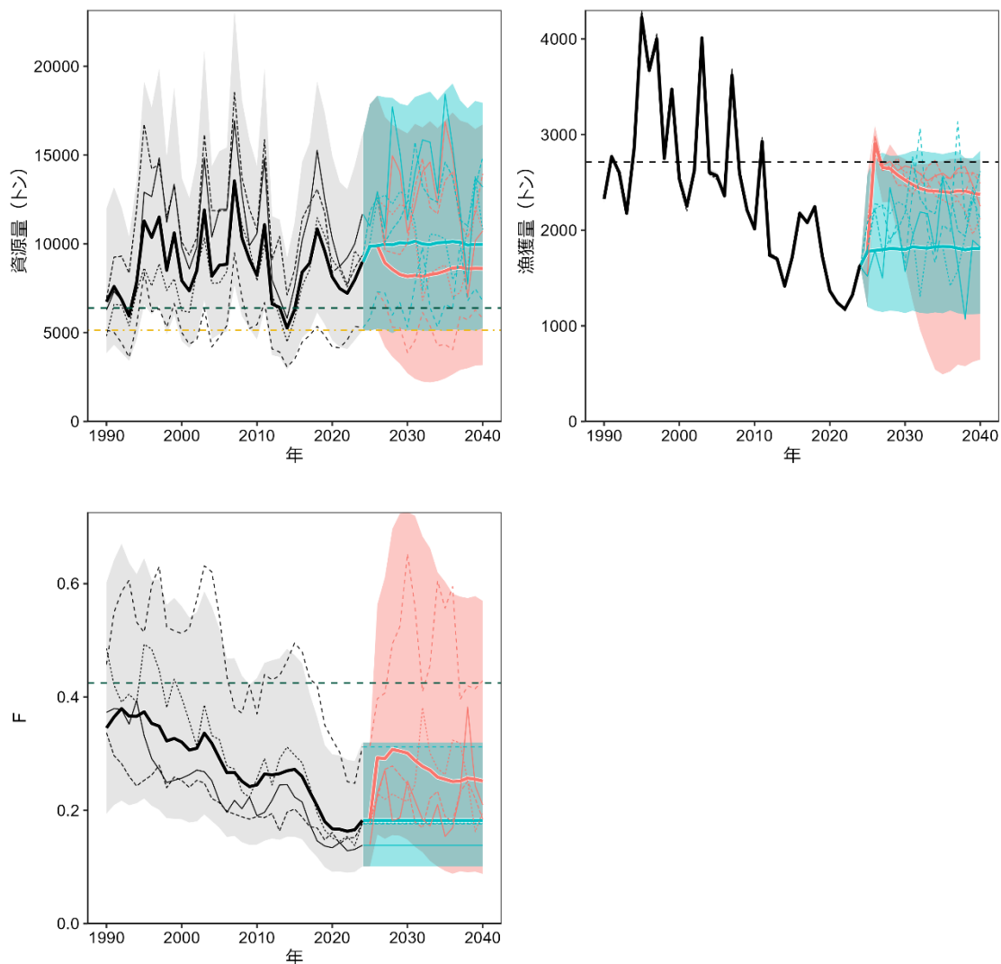
補足図 5-2. 余剰生産モデルで推定されたパラメータと漁獲管理規則案に基づいて予測された将来の資源量、漁獲圧および漁獲量 青色の太い実線と網掛けは現状の漁獲圧 (F2024) で、赤色の太い実線と網掛けは調整係数 \beta=0.7 とする漁獲管理規則案で漁獲した場合の予測された値の中央値と 90%予測区間、黒の太い実線と灰色の網掛けは 1990~2024 年漁期に推定された値の中央値と 90%信頼区間、各色の細い線は反復計算の結果の例示である。資源量の図に示された緑色の破線は目標管理基準値案を達成する水準、黄色の一点鎖線は限界管理基準値案の水準である。漁獲量の図に示された黒色の破線は MSY 水準、漁獲圧 (F) の図に示された緑色の破線は Fmsy 水準である。
