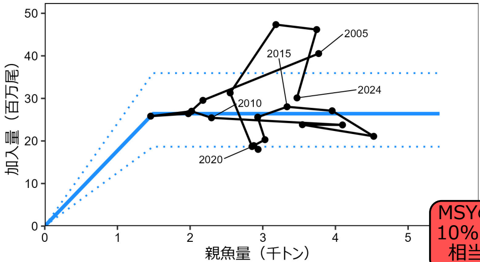
図4 再生産関係
