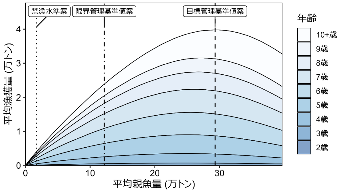
図3. 管理基準値案および禁漁水準案と年齢別漁獲量曲線の関係 (SC 補足図 3-2) 将来予測シミュレーションにおける平衡状態での、親魚量に対する年齢別漁獲量の平均値と、それぞれの管理基準値案の位置関係を示す。漁業がなかった場合を仮定した初期親魚量 (SB0) は 56.7 万トンである。
