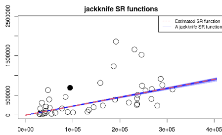
a) 最小二乘法（自己相関なし）
