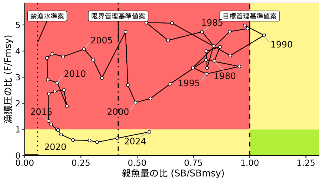
図4. 神戸プロット (SC 補足図 3-1) 縦軸は各年の漁獲圧 F の F_{msy} との比である。図中の目標管理基準値案、限界管理基準値案、および禁漁水準案には、それぞれ SB_{msy} 、 SB_{0.6msy} 、および SB_{0.1msy} を用いた。
