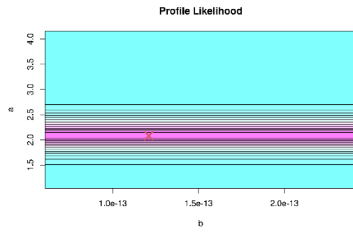
d) 最小二乗法（二段階推定）
