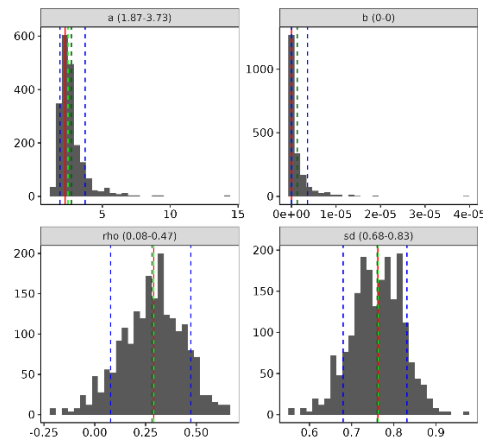
d) 最小二乗法 (二段階推定)
