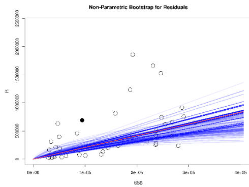
c) 最小二乗法（自己相関なし）
