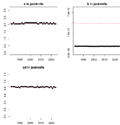
a) 最小絶対値法（自己相関なし）
