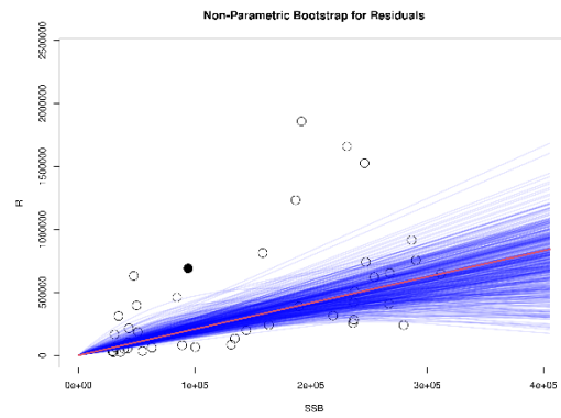
d) 最小二乗法（二段階推定）
