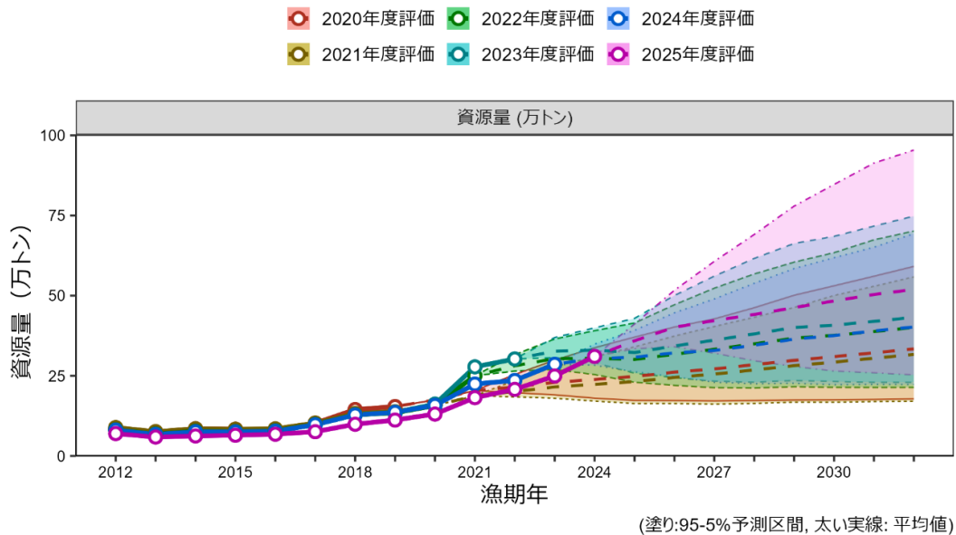
補足図 10-2. 評価年度別の資源量の比較
