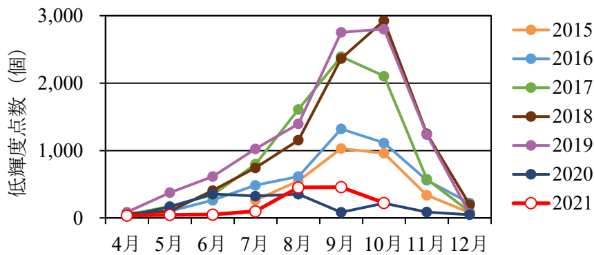
補足図 4-3. 東経 130～137 度、北緯 38 度 37 分～北緯 43 度 (2018 年 8 月以降は東経 130～138 度 30 分、北緯 38 度 37 分～北緯 45 度。北朝鮮水域、ロシア水域、我が国 EEZ を含む) の海域における低輝度点 ( 300 \times 10^{-10} \text{ W cm}^{-2} \text{ sr}^{-1} 未満、補足図 4-1 の水色～青色の点) の日々のカウント数の月間最大値の推移。光点の多くは北朝鮮漁船で、中国の 2 そうびき網船等も含まれると推察される。
