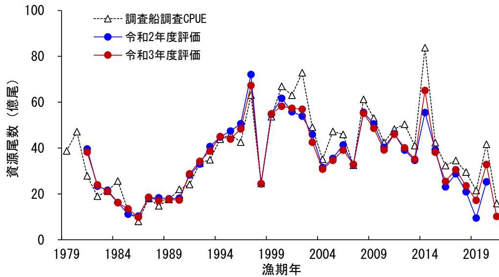
補足図 2-2. 補足図 2-1 に示す各指標値から推定された資源尾数の推移
