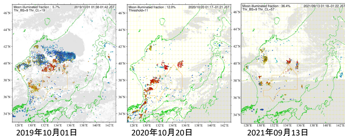
補足図 4-1. 日本海の NPP 衛星夜間可視データから抽出された光点の分布 2019~2021 年の比較。暖色系は高輝度点、寒色系は低輝度点、灰色は雲域を示す。
