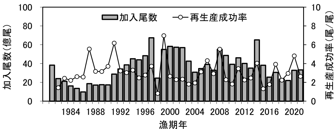
図 4-5. 加入尾数と再生産成功率 (RPS) の推移 スルメイカでは、加入尾数と資源尾数とは同義である。
