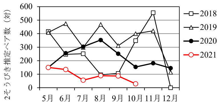
補足図 4-5. 東経 130～134 度、北緯 38～42 度（北朝鮮水域、ロシア水域、我が国 EEZ を含む）の海域において ALOS-2/PALSAR-2 の衛星画像解析により 2 人組と推定された漁船のペア数の推移。2 人組船であるため、漁船数はペア数の 2 倍。
