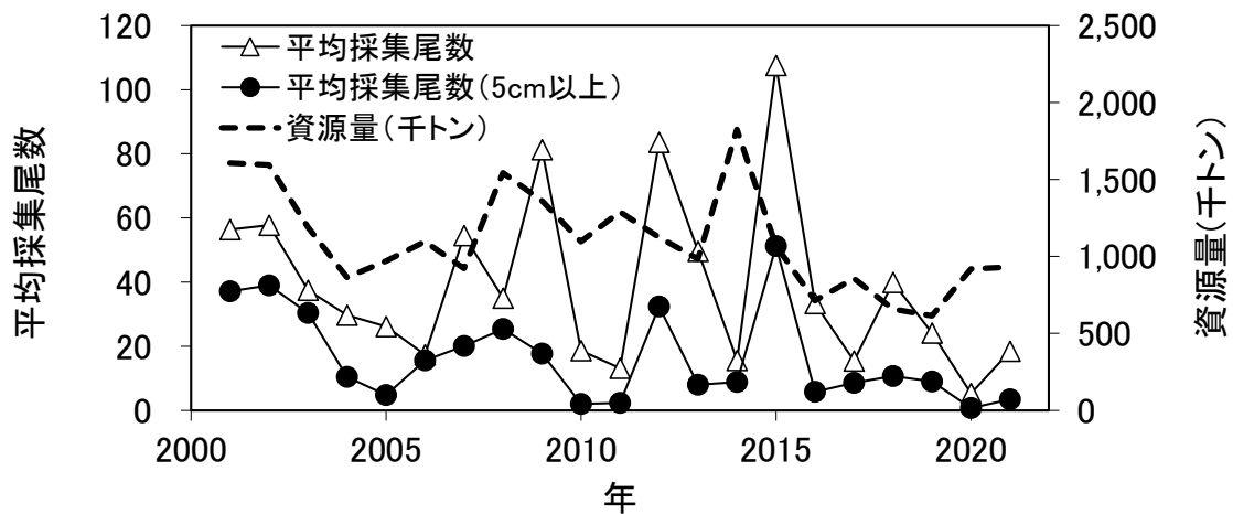
補足図 3-8. 新規加入量調査の平均採集尾数と資源量の経年変化
