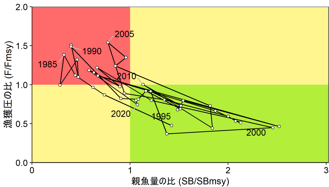
図 4-9. 最大持続生産量 MSY を実現する親魚量(SBmsy)と MSY を実現する漁獲圧(Fmsy) に対する、過去の親魚量および漁獲圧の関係（神戸プロット）
