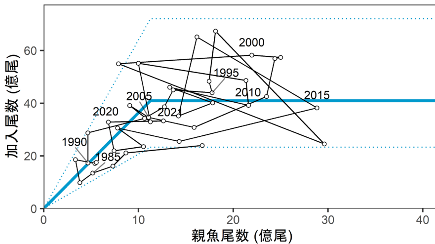
図 4-8. 親魚量と加入量の関係（再生産関係） 令和 2 年 7 月に開催された「管理基準値等に関する研究機関会議」（久保田ほか 2020a）で提案された再生産関係式 青実線は再生産関係。再生産関係の上下の点線は、仮定されている再生産関係において観察データの 90%が含まれると推定される範囲である。図中の数字は年級群を示す。2021 年漁期の親魚尾数は F2021（予測値）による漁獲後の残存資源尾数の推定値。
