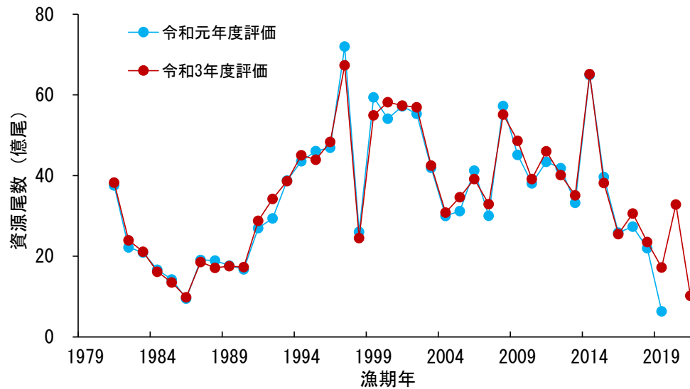
補足図 2-3. 令和元年度評価および今年度評価での標準化 CPUE から推定された資源尾数の推移
