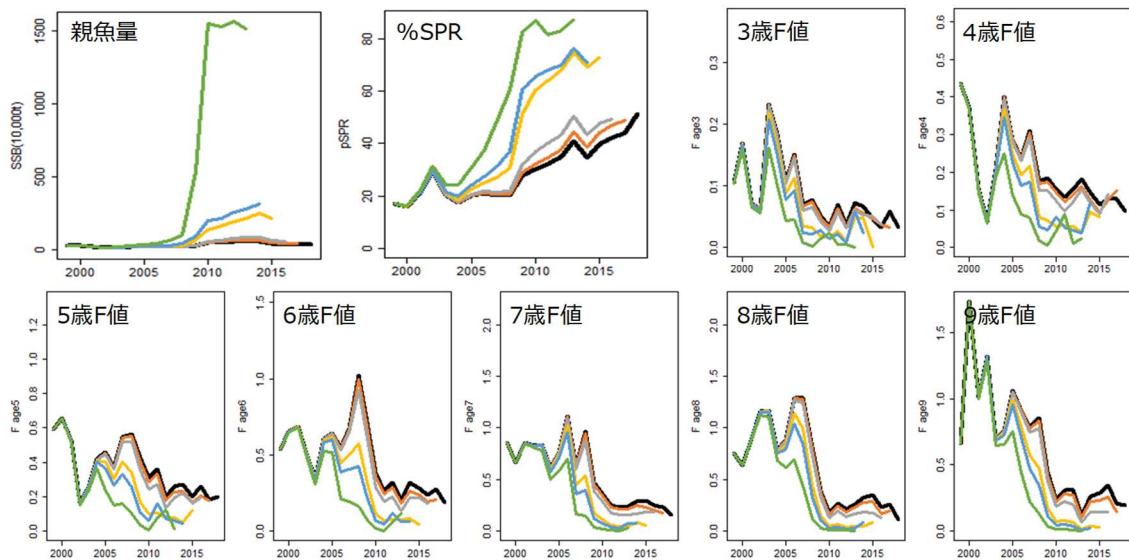
補足図 6-1. リッジ VPA のペナルティによるレトロスペクティブ解析結果の比較 (続き)
