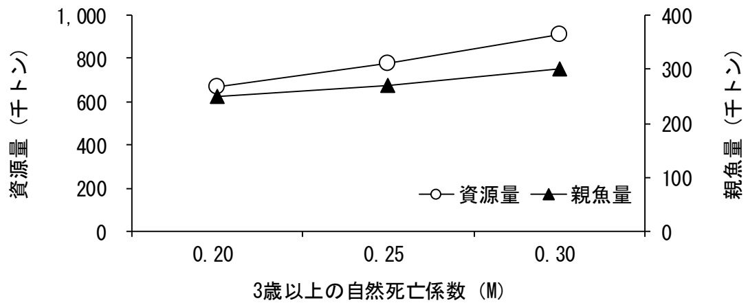
図 4-8. 資源量と親魚量に対する自然死亡係数 M の影響 (2018 年漁期の資源量と親魚量)
