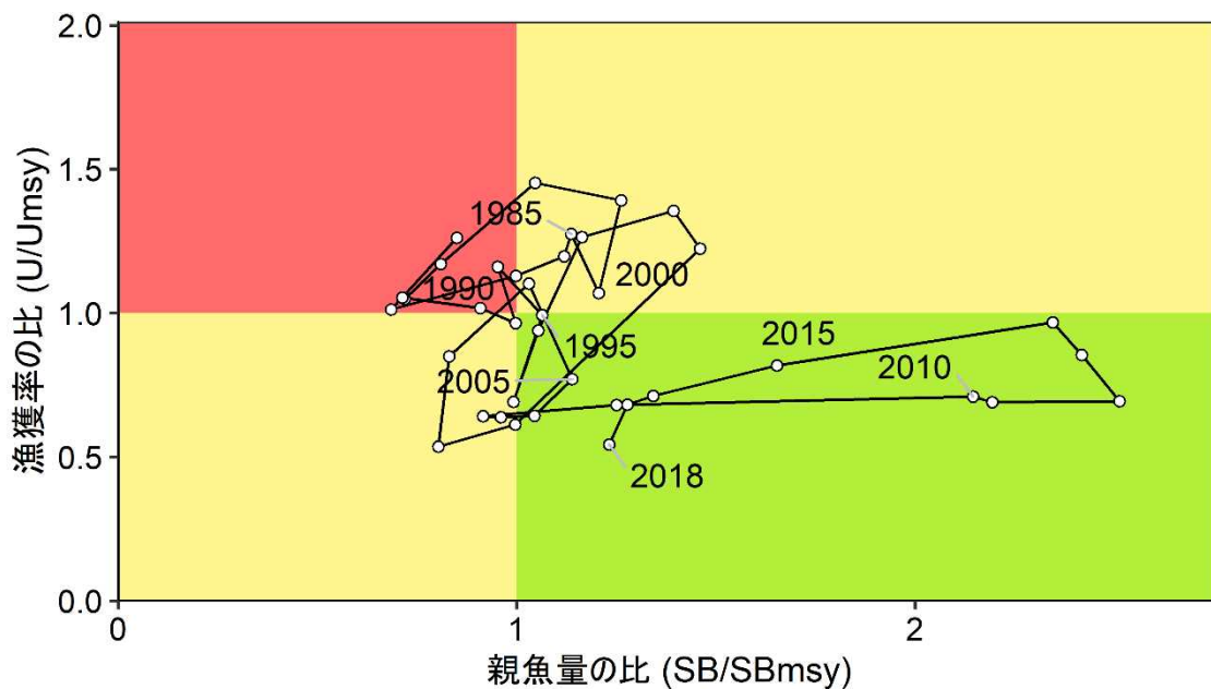
補足図 7. 最大持続生産量 (MSY) を実現する親魚量 (SBmsy) および MSY を実現する漁獲割合 (Umsy) に対する、親魚量および漁獲割合の関係 (神戸プロット)
