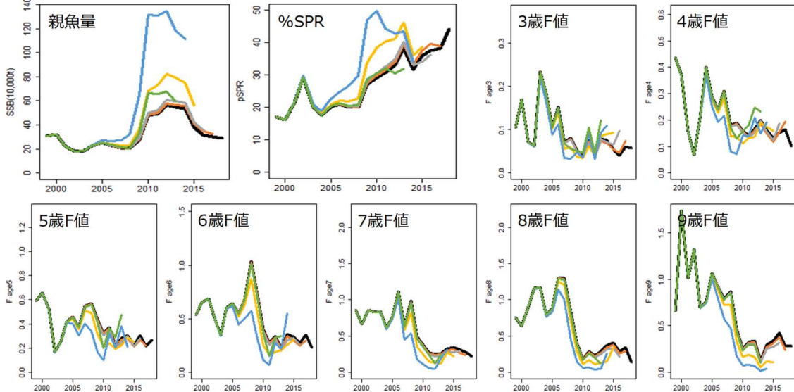
補足図 6-1. リッジ VPA のペナルティによるレトロスペクティブ解析結果の比較 (続き) すべての年齢の F 値の二乗値に一律にペナルティ \lambda を与えて親魚量のレトロスペクティブバイアスを最小とした場合 (上段) と、同様にペナルティ \lambda を与えて %SPR のレトロスペクティブバイアスを最小とした場合 (下段)
