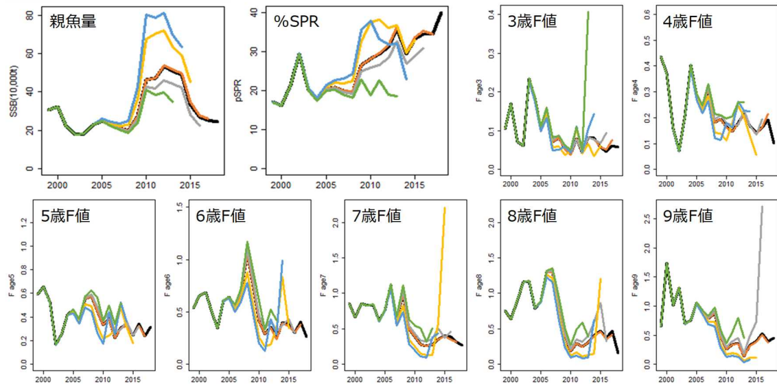
補足図 6-1. リッジ VPA のペナルティによるレトロスペクティブ解析結果の比較 ペナルティを与えなかった場合 ( \lambda=0 ) の例を示す。
