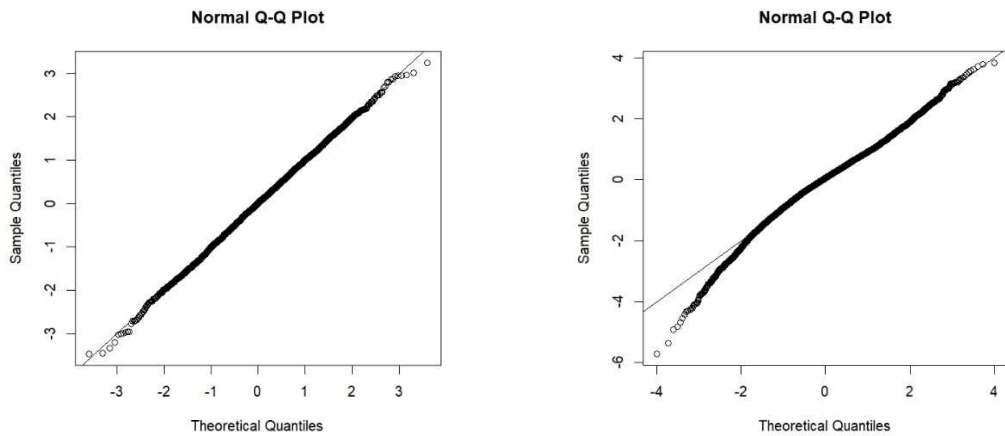
補足図 5-2. モデルの残差 (Randomized Quantile Residuals) の QQ プロット 左は第 1 段階、右は第 2 段階のモデルである。図の縦軸は残差の値、横軸は残差の期待値を示す。
