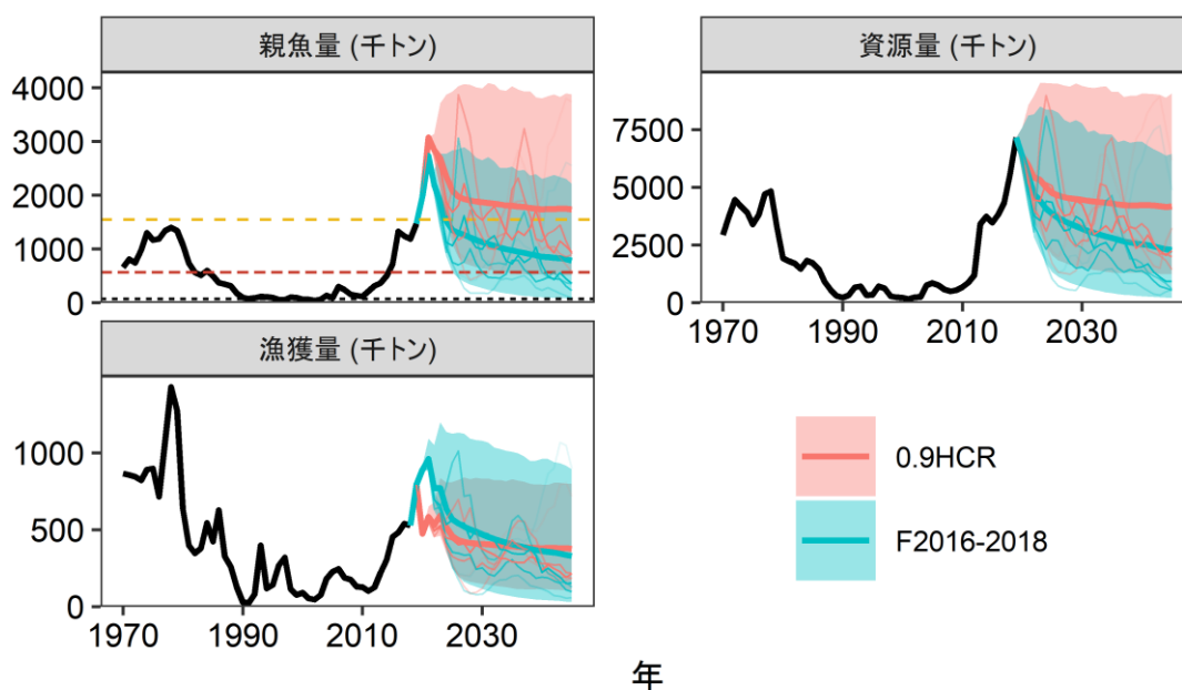
補足図 8-2. 漁獲管理規則案 (HCR) を用いた場合の将来予測と F2016-2018 で漁獲を続けた場合の将来予測の比較 太実線は平均値、網掛けは 80%信頼区間、細線は 3 通りの将来予測の例示である。親魚量の図の黄破線は目標管理基準値案、赤点線は限界管理基準値案、黒点線は禁漁水準案を示す。2019 年漁期の漁獲量は現状の漁獲圧 (F2016-2018) から予測される 794 千トン。漁獲管理規則案の \beta は 0.9 のものを示す。F2016-2018 は、 F_{msy} と等しい選択率において推定される %SPR が 2016~2018 年漁期の平均 F 値から推定される %SPR と等しくなる値とした。
