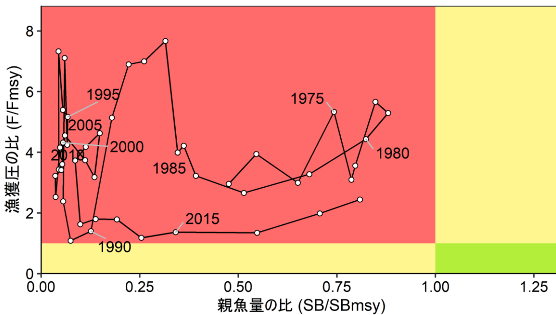
図 4-13. 最大持続生産量 MSY を実現する親魚量 (SBmsy) と漁獲圧 (Fmsy) に対する、過去の親魚量および漁獲圧の関係（神戸プロット） 漁獲圧と親魚量の値は 3 年移動平均値。2015 は 2013～2015 年漁期の平均値を示す。
