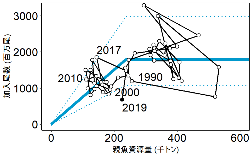
図 4-11. 親魚量と加入量の関係（再生産関係） 平成 31 年 4 月に開催された「管理基準値等に関する研究機関会議」（安田ほか 2019）で提案された再生産関係式（実線）。丸印は実測データ（1973~2019）であり、2019 年の値は●で示す。点線は仮定されている再生産関係において観察データの 90%が含まれると推定される範囲である。
