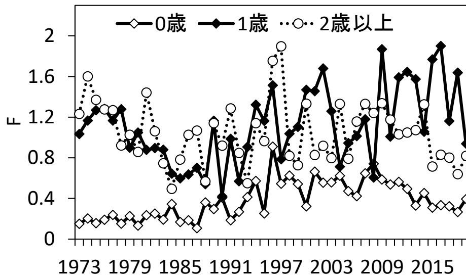
図 4-7. 年齢別漁獲係数 F の推移
