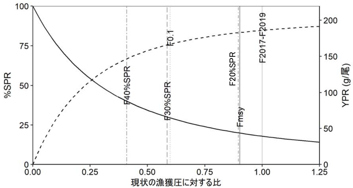
図 4-10. 現状の漁獲圧（F2017-2019）に対する YPR と%SPR の関係
