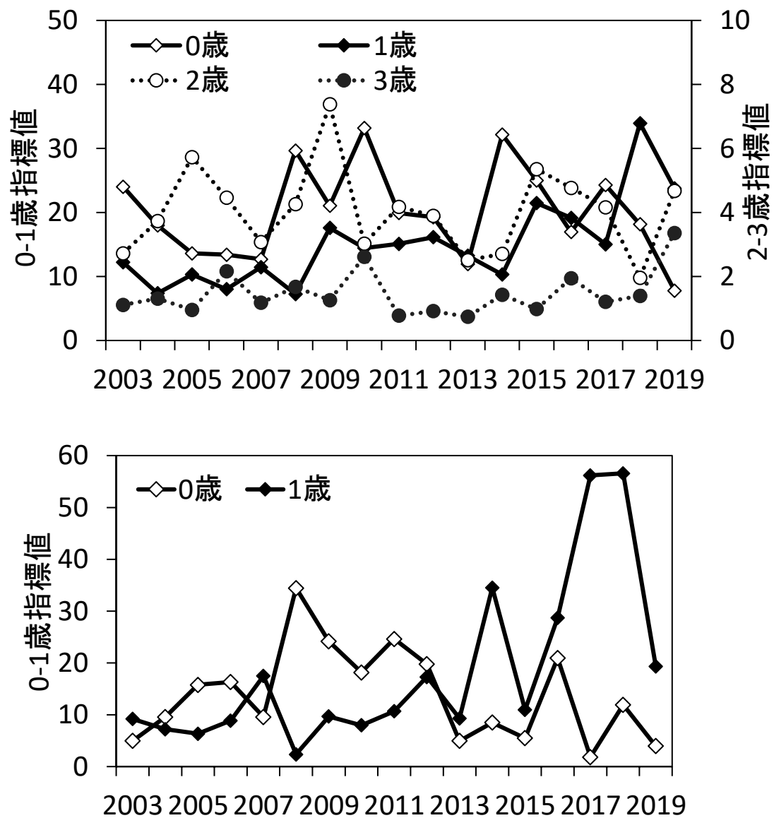
図 4-1. 東シナ海・日本海西部で操業する大中型まき網の銘柄別漁獲量から算出した年齢別の資源量指標値の推移（上図）と境港港に水揚げする中型まき網の豆銘柄の漁獲量と入港隻数から算定した 0 歳と 1 歳の資源量指標値の推移（下図）。
