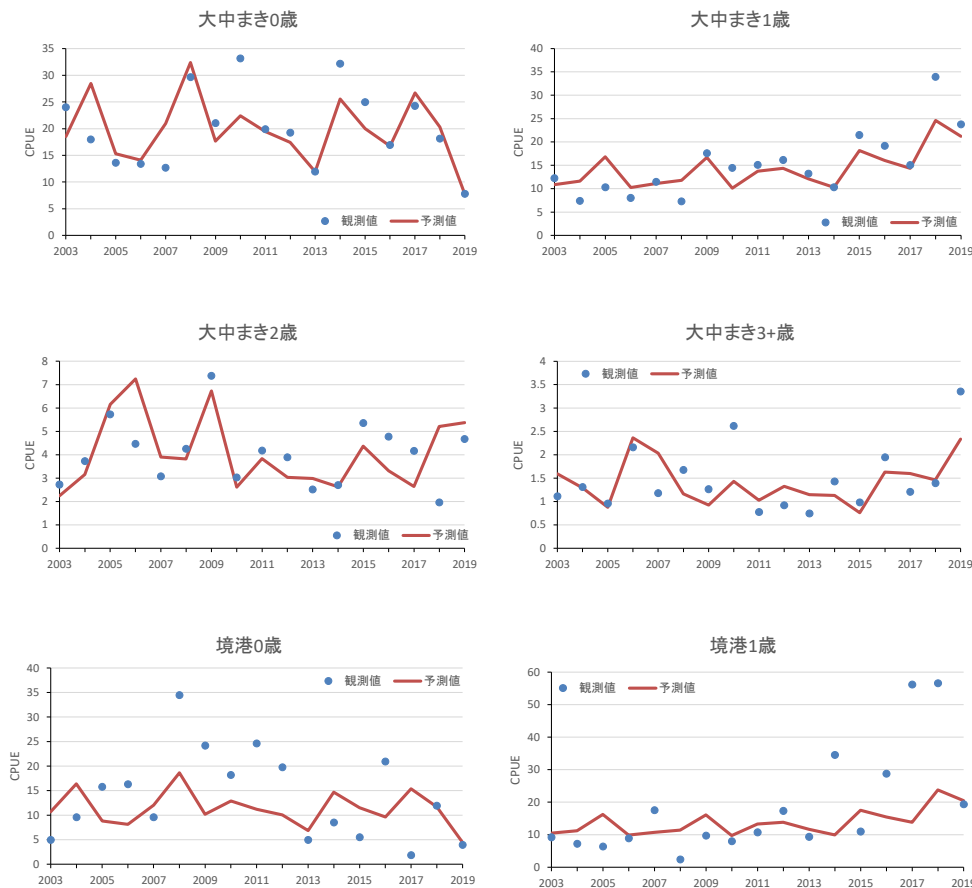
補足図 2-1 指標値の観測値とモデルの予測値
