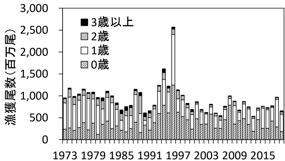
図 3-2. 年齢別漁獲尾数の推移
