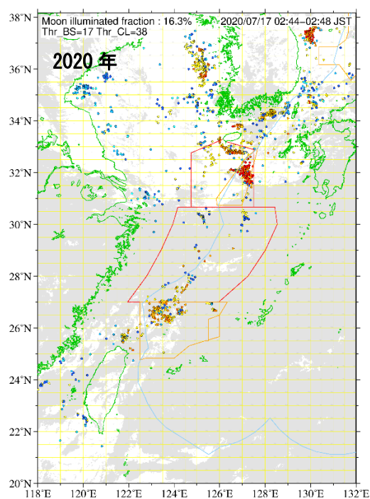
補足図 7-1. 2014～2020 年 7 月の東シナ海における人工衛星夜間可視データから抽出された操業点（続き）
