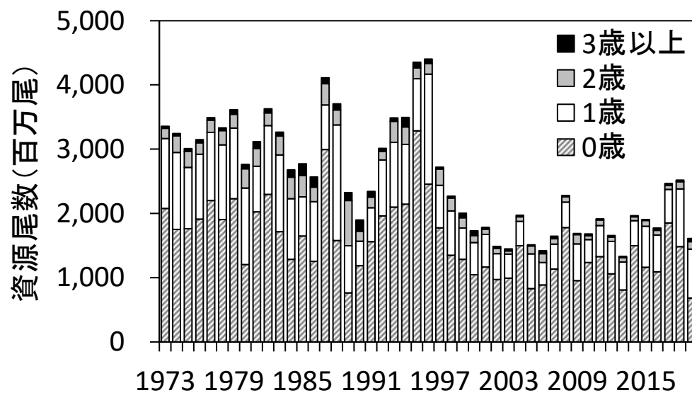
図 4-3. 年齢別資源尾数の推移
