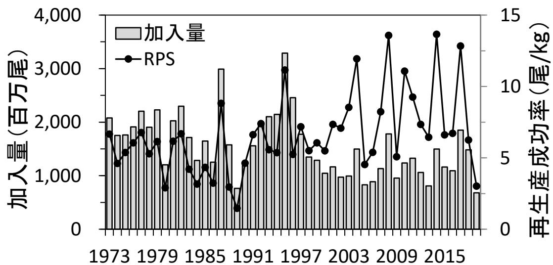
図 4-5. 加入量と再生産成功率 (RPS: 尾/kg) の推移
