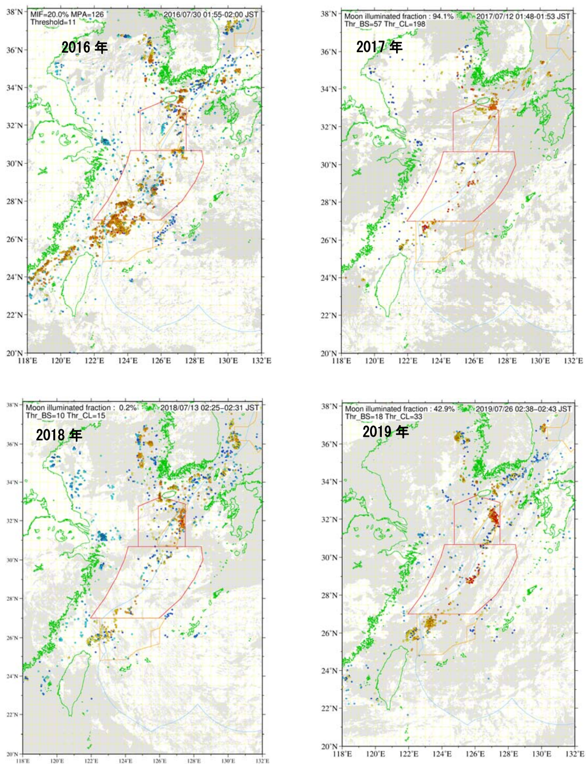
補足図 7-1. 2014～2020 年 7 月の東シナ海における人工衛星夜間可視データから抽出された操業点（続き）
