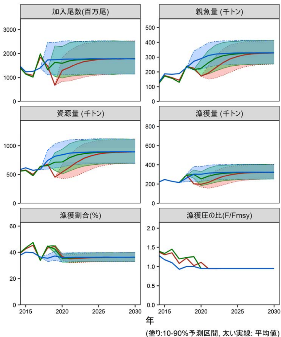
補足図 8-1. 加入尾数、資源量、親魚量、漁獲量、漁獲割合、漁獲圧の比の将来予測結果 （青：2018 年度資源評価に基づく研究機関会議予測、緑：2019 年度資源評価、赤：今年度資源評価。いずれも \beta=0.95 の時。）
