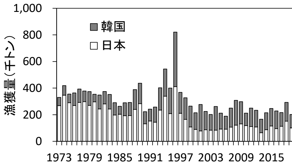
図 3-1. 漁獲量の推移
