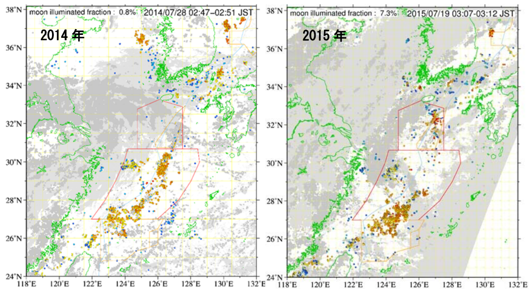
補足図 7-1. 2014～2020 年 7 月の東シナ海における人工衛星夜間可視データから抽出された操業点
