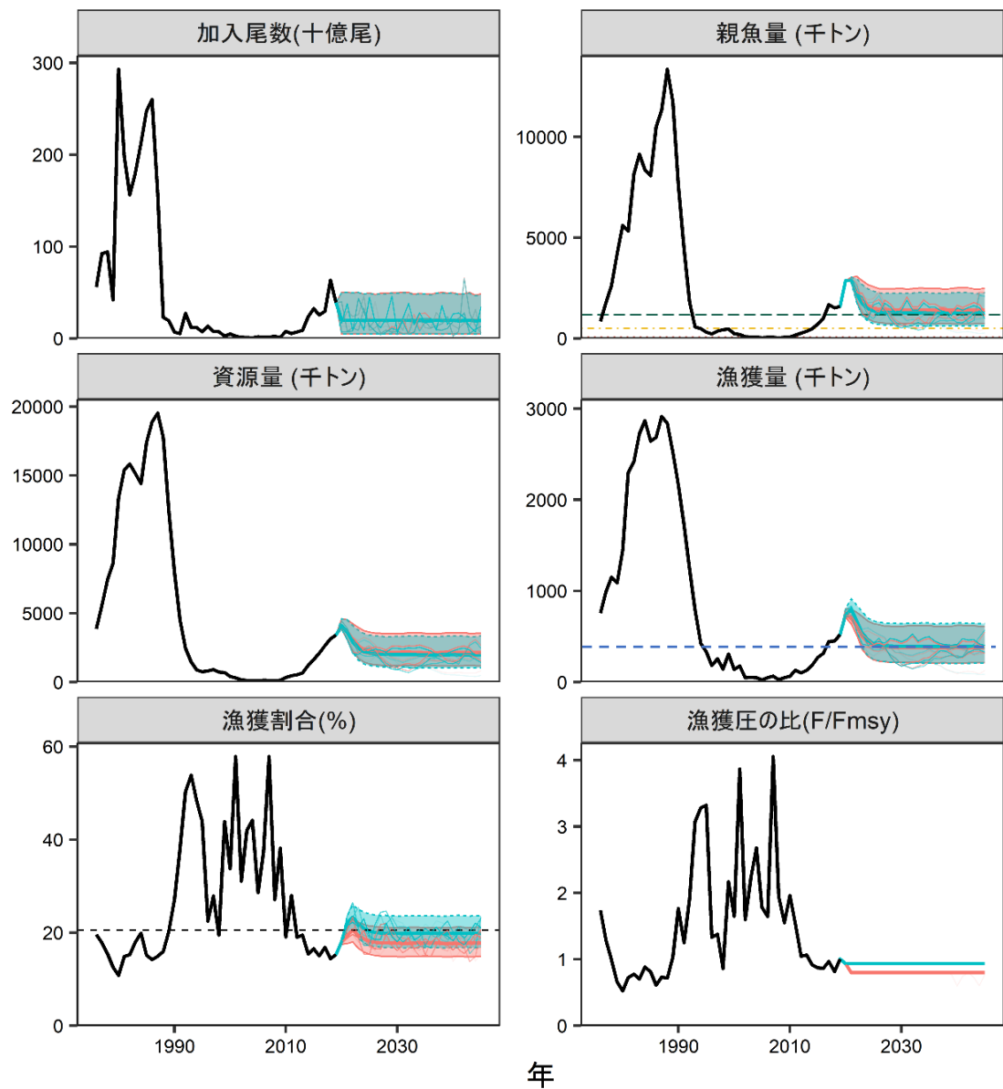
補足図 6-2. 管理基準値案に基づく漁獲管理規則案を用いた将来予測(赤色)と現状の漁獲圧で漁獲を続けた場合の将来予測(緑色)
