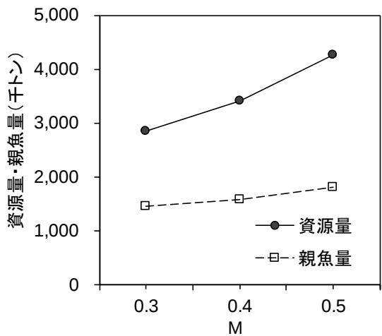
図 4-5. 自然死亡率 M と資源量、親魚量の関係 M の変化に対する 2019 年の推定値の感度解析。
