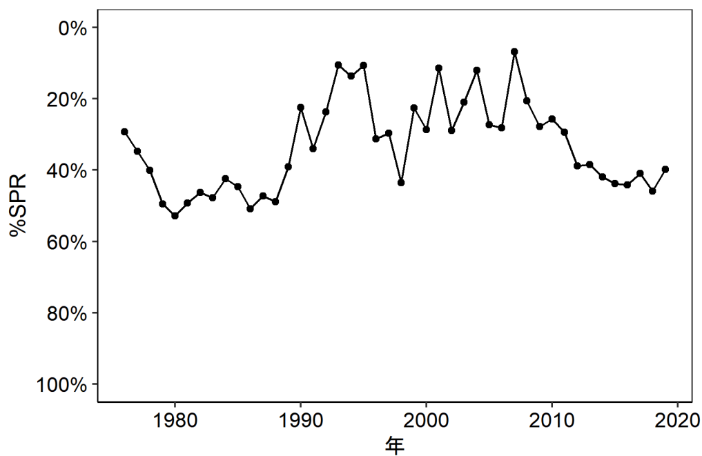
図 4-6. %SPR 値の推移 %SPR は、漁獲がないときの親魚量に対する漁獲があるときの親魚量の割合を示し、F が高い（低い）と %SPR は小さく（大きく）なる。
