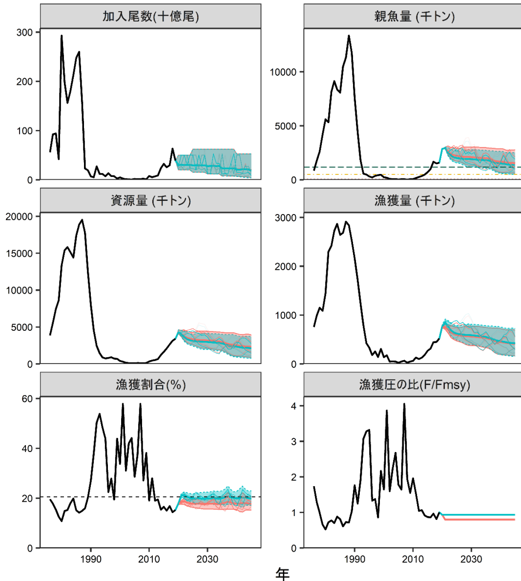
補足図 8-2. 加入量の誤差に残差のバックワードリサンプリングを適用した場合における、管理基準値案に基づく漁獲管理規則案を用いた将来予測(赤色)と現状の漁獲圧で漁獲を続けた場合の将来予測(緑色) 太実線は平均値、網掛けはシミュレーション結果の90%が含まれる90%予測区間、細線は3通りの将来予測の例示である。親魚量の図の緑破線は目標管理基準値案、黄点線は限界管理基準値案を示す。漁獲割合の図の破線は U_{msy} を示す。安全係数 \beta には0.8を用いた。
