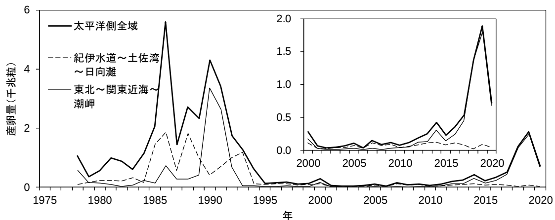
図 4-1. 産卵量の推移 卵稚仔調査協会による前年 10 月から 9 月までの集計値 2020 年は 5 月までの暫定値。太平洋側全域は同協会の区分の海区 I ～IV、紀伊水道～土佐湾～日向灘は海区 III、東北～関東近海～潮岬は海区 I・II の値。
