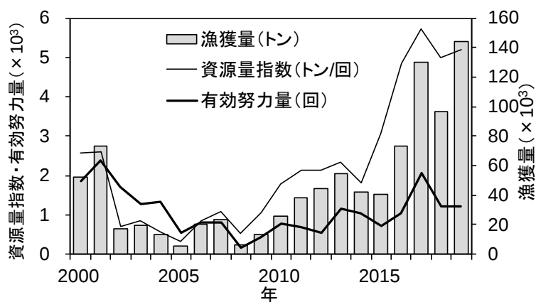
図 3-3. 北部まき網の有効努力量と漁獲量、資源量指数の推移 (JAFIC 集計値、道東含まず) 努力量＝投網数、資源量指数＝ \sum 緯度経度 30 分単位メッシュの CPUE、有効努力量＝漁獲量／資源密度指数、資源密度指数＝資源量指数／有漁メッシュ数。
