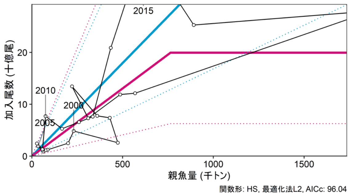
図 1. 再生産関係
