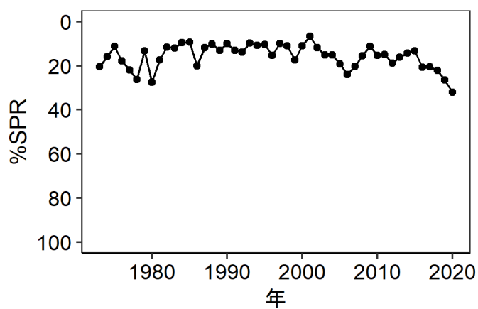
図 4-10. %SPR 値の推移
