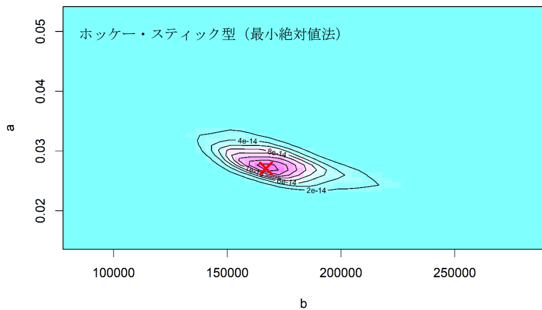
補足図 1-8. HS 型再生産関係における推定パラメータのプロファイル尤度 ×印は推定されたパラメータ値における尤度に相当する。
