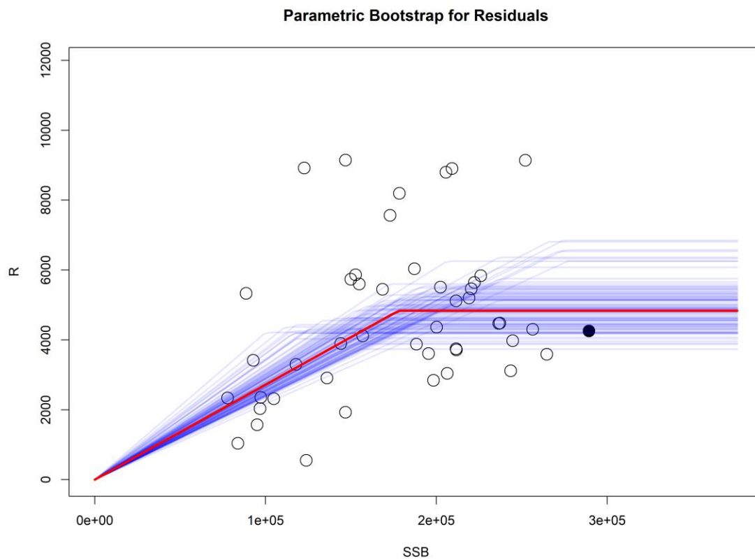
補足図 1-6. HS 型再生産関係における残差ブートストラップ解析の結果 赤線は元データでの推定値、青線はパラメトリックブートストラップでの推定値である。横軸は親魚量（トン）、縦軸は加入量（百万尾）である。丸印は分析に使用した親魚量と加入量のプロットであり、黒丸は使用したデータ期間の最終年（2017 年）を示す。
