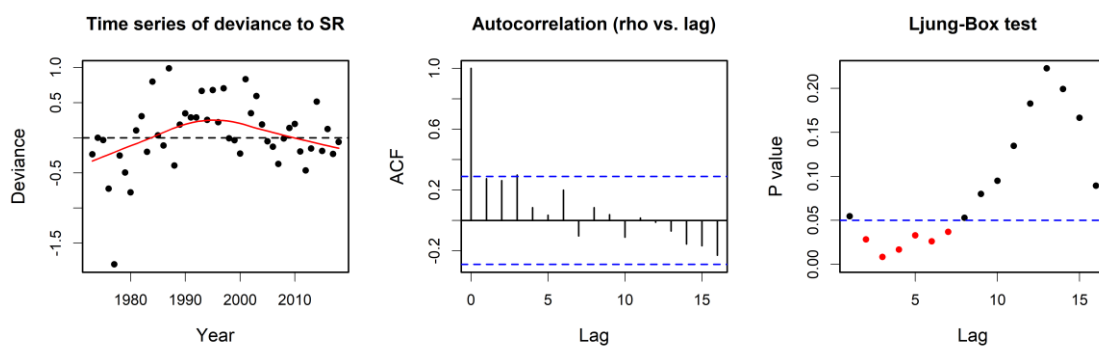
補足図 1-2. HS 型再生産関係における（左）標準化残差の時系列トレンド、（中央）コレログラム、（右）Ljung-Box 検定における P 値
