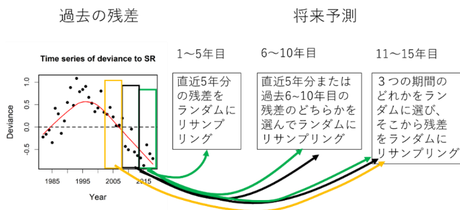
補足図 6-1. バックワードリサンプリングの概念図
