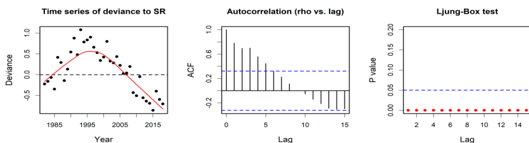
補足図 1-2. HS 型および RI 型再生産関係における（左）標準化残差の時系列トレンド、（中央）コレログラム、（右）Ljung-Box 検定における P 値
