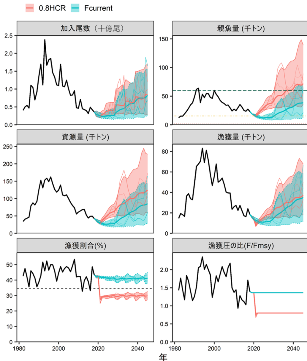
補足図 6-2. シナリオ①で漁獲管理規則案を用いた将来予測（赤色）と現状の漁獲圧で漁獲を続けた場合の将来予測（緑色）の比較
