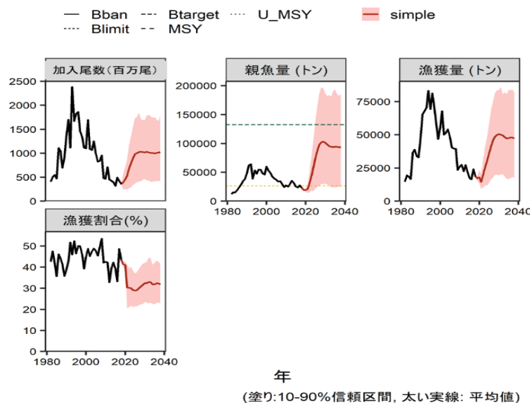
補足図 4-2. シナリオ②の MSE 将来予測（真の再生産関係が BH 型と仮定し、RI 型の漁獲管理規則案を用いた場合） 太実線は平均値、網掛けはシミュレーション結果の 80%が含まれる 80%予測区間。親魚量の図の破線は BH 型の管理基準値案（緑：目標管理基準値案、黄：限界管理基準値案）。2019 年と 2020 年の漁獲量は予測される資源量と F_{\text{current}} により仮定し、2021 年以降の漁獲は漁獲管理規則案に基づく（図 5）。安全係数 \beta には 0.8 を用いた。
