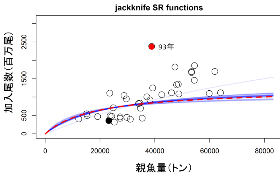
補足図 1-4. RI 型および BH 型の再生産関係で自己相関を同時推定した場合のジャックナイフ解析での推定結果
