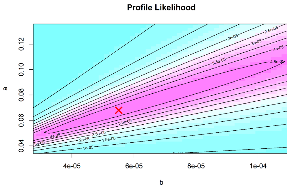
補足図 1-8. RI 型および BH 型の再生産関係で自己相関を同時推定した場合の推定パラメータのプロファイル尤度 ×印は最尤推定されたパラメータ値。
