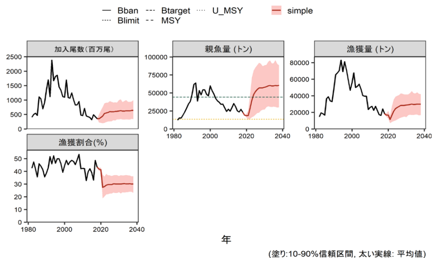
補足図 4-3. シナリオ③の MSE 将来予測（再生産関係が RI 型と仮定し、重み付き平均モデルの漁獲管理規則案を用いた場合） 太実線は平均値、網掛けはシミュレーション結果の 80%が含まれる 80%予測区間。親魚量の図の破線は RI 型の管理基準値案（緑：目標管理基準値案、黄：限界管理基準値案）。2019 年と 2020 年の漁獲量は予測される資源量と F_{current} により仮定し、2021 年以降の漁獲は漁獲管理規則案に基づく（図 5）。安全係数 \beta には 0.8 を用いた。
