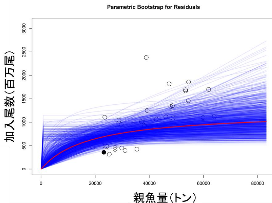
補足図 1-6. RI 型および BH 型の再生産関係で自己相関を同時推定した場合の残差ブートストラップ解析の結果
