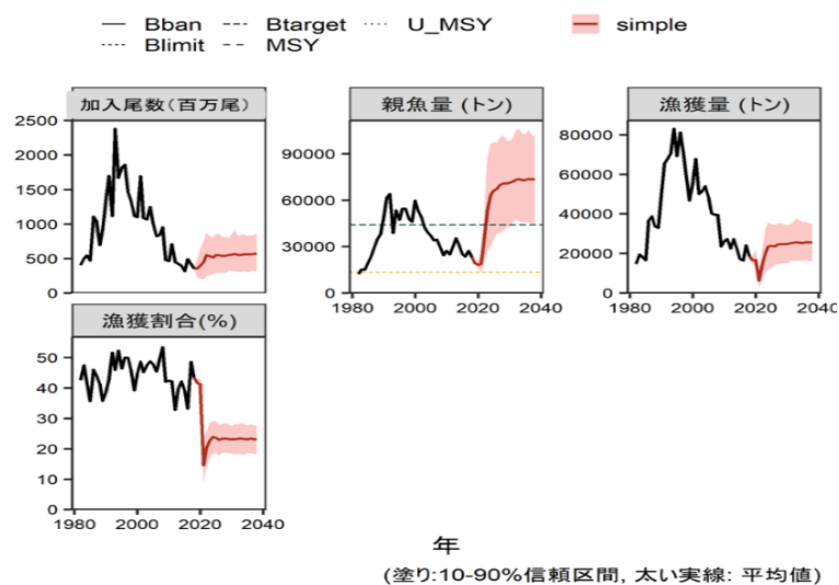
補足図 4-1. シナリオ①の MSE 将来予測（真の再生産関係が RI 型と仮定し、BH 型の漁獲管理規則案を用いた場合） 太実線は平均値、網掛けはシミュレーション結果の 80%が含まれる 80%予測区間。親魚量の図の破線は RI 型の管理基準値案（緑：目標管理基準値案、黄：限界管理基準値案）。2019 年と 2020 年の漁獲量は予測される資源量と F_{\text{current}} により仮定し、2021 年以降の漁獲は漁獲管理規則案に基づく（図 5）。安全係数 \beta には 0.8 を用いた。
