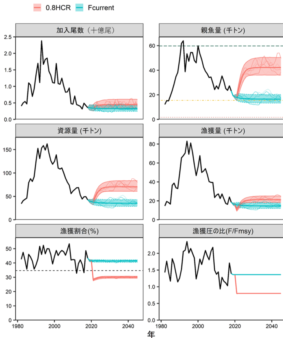
補足図 6-3. シナリオ②で漁獲管理規則案を用いた将来予測（赤色）と現状の漁獲圧で漁獲を続けた場合の将来予測（緑色）の比較
