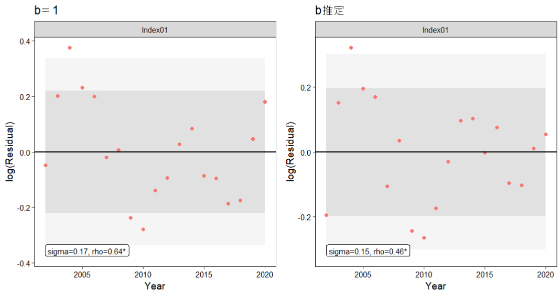
補足図 4-2. b=1 とした場合 (左) および b を推定した場合 (右) の残差プロット 濃い灰色が 80%、薄い色が 95%の信頼区間を示す
