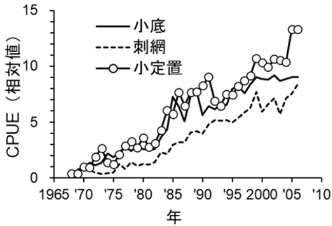
図 7. 農林水産統計による瀬戸内海区の小底、刺網、小定置の CPUE の推移（2006 年まで） 1970 年を 1 とした。
