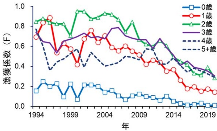
図 11. 年齢別漁獲係数 F の推移
