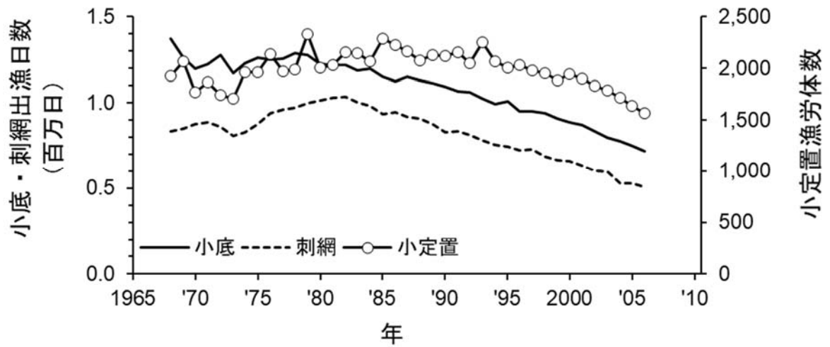
図 5. 農林水産統計による瀬戸内海区の小底、刺網、小定置の努力量の推移 (2006 年まで)
