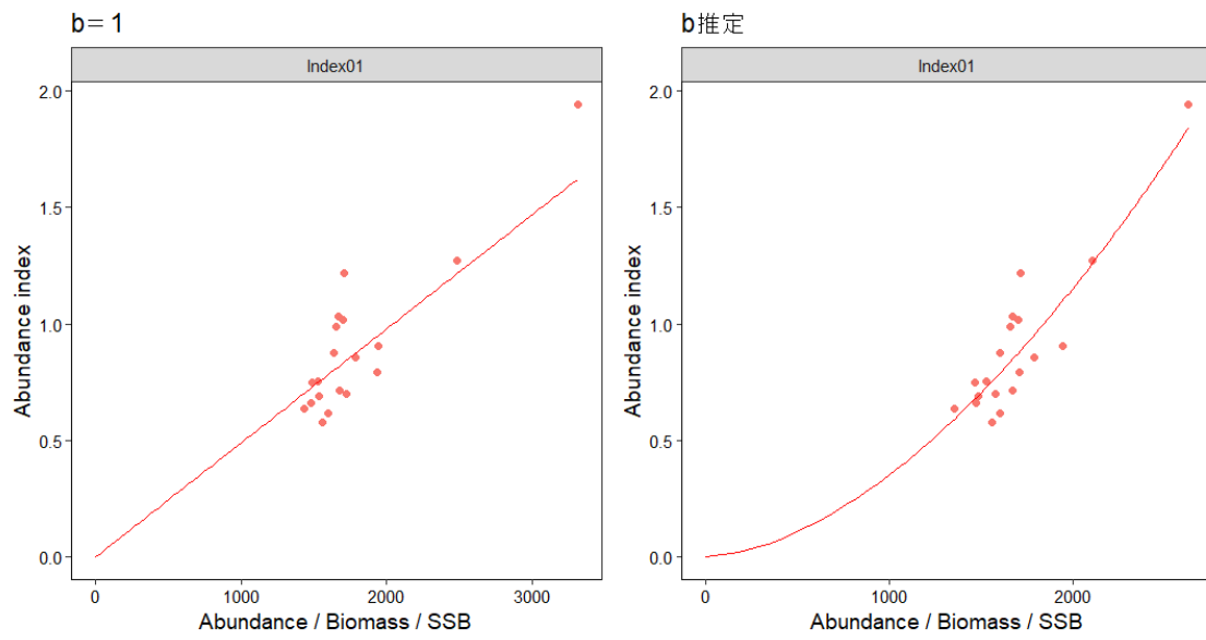
補足図 4-4. 漁獲対象資源とチューニング指標値の対応 (左 : b=1 、右 : b を推定)
