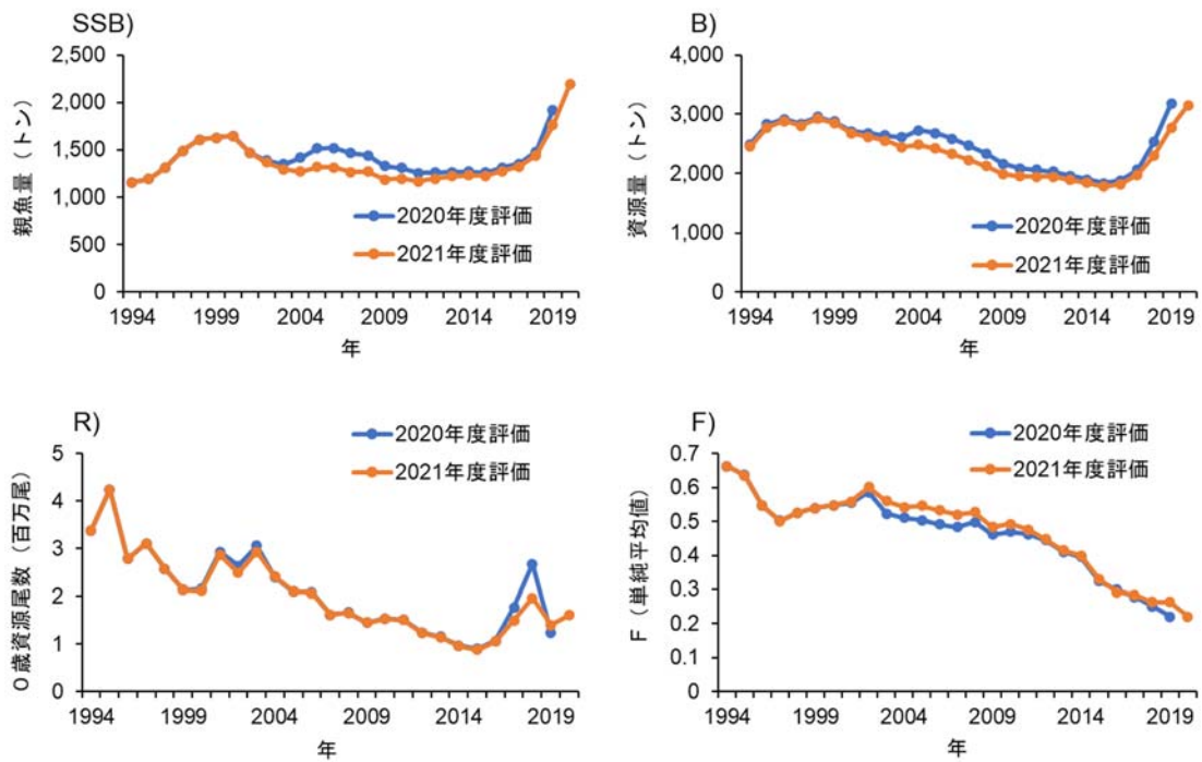
補足図 2-3. 親魚量 (SSB)、資源量 (B)、0 歳資源尾数 (R)、漁獲係数 (F、単純平均値) の 2020 年度資源評価結果との差異 (青線が 2020 年度資源評価結果、赤線が本年度資源評価結果を示す)。
