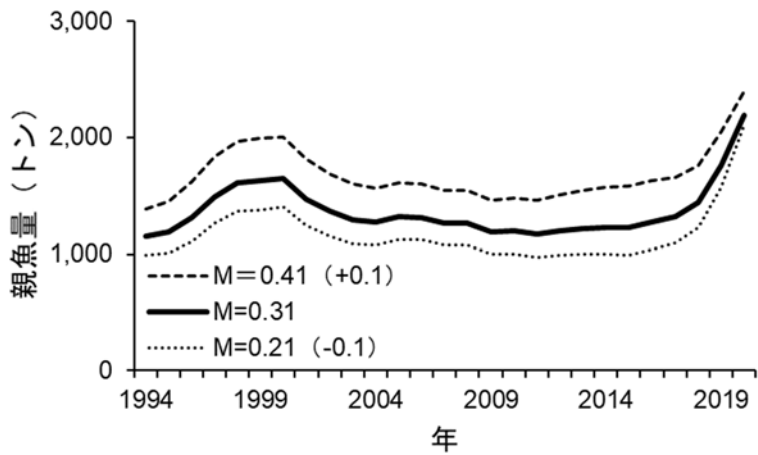
図 17. 自然死亡係数 M の値による親魚量の感度解析
