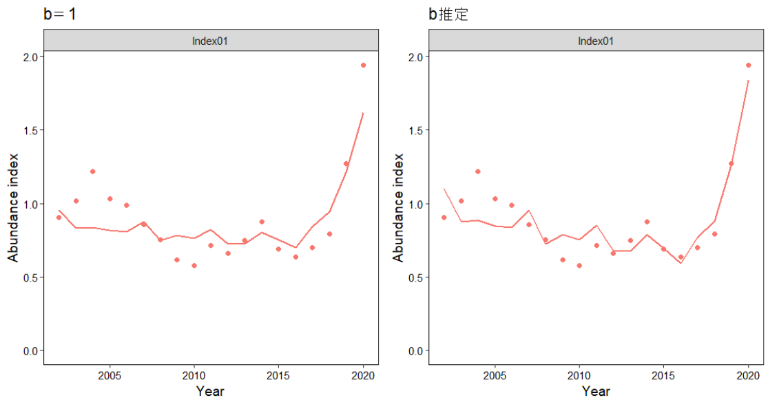
補足図 4-3. チューニング指標値と漁獲対象資源の推移 (左 : b=1 、右 : b を推定)
