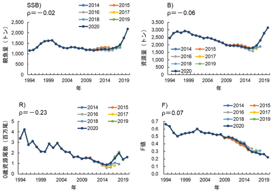
補足図 2-2. 親魚量 (SSB)、資源量 (B)、0歳資源尾数 (R)、漁獲係数 (F) のレトロスペクティブ解析結果 Fは全年齢の単純平均値、凡例の数字は VPA 最終年を示す。
