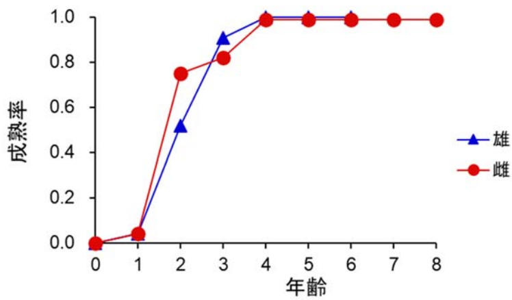
図3. 雌雄別年齢別成熟割合
