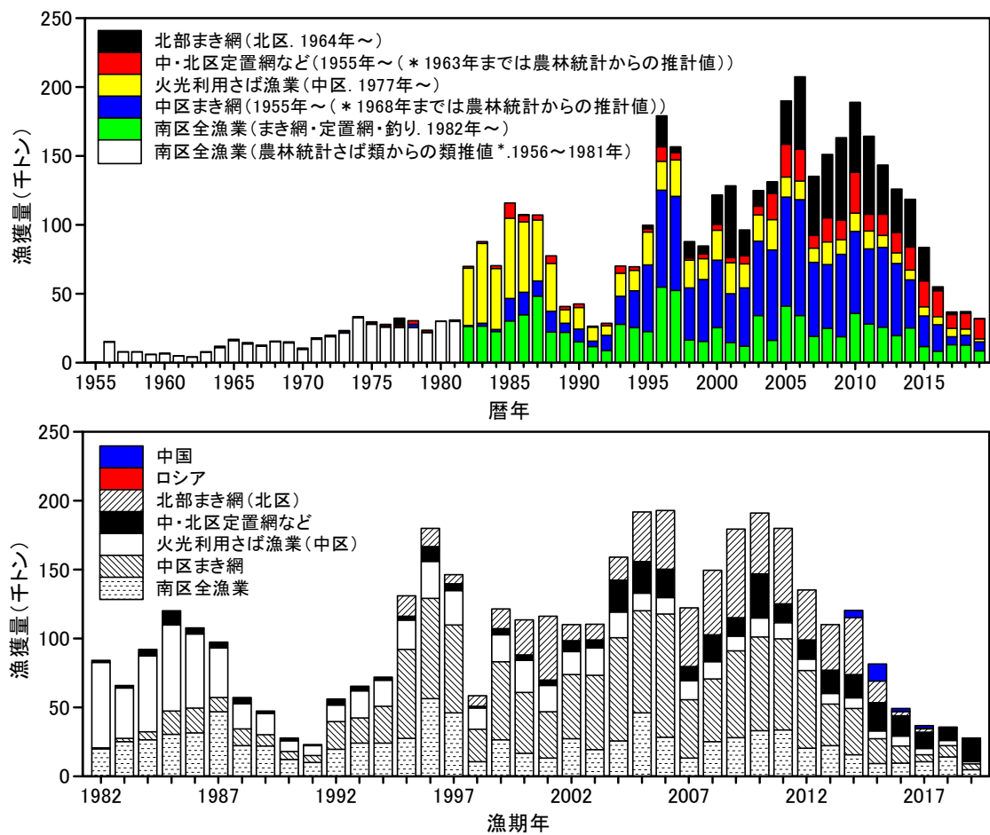
図 3-1. 漁獲量の推移 太平洋側の暦年(1～12月、日本のみ、上図)および漁期年(7月～翌年6月、外国を含む、下図)別の海区・漁業種類別漁獲量。*南区の1982～2005年の農林水産統計さば類漁獲量に対する主要港ゴマサバ水揚げ量(各県資料)の比率を使って求めた。下図の2014年漁期以降の中国およびロシアの漁獲量は推定値。
