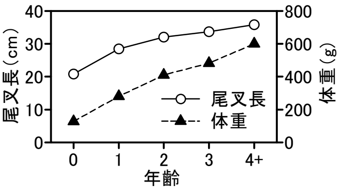
図 2-2. 年齢と成長 (2015～2019 年漁期漁獲物の平均)
