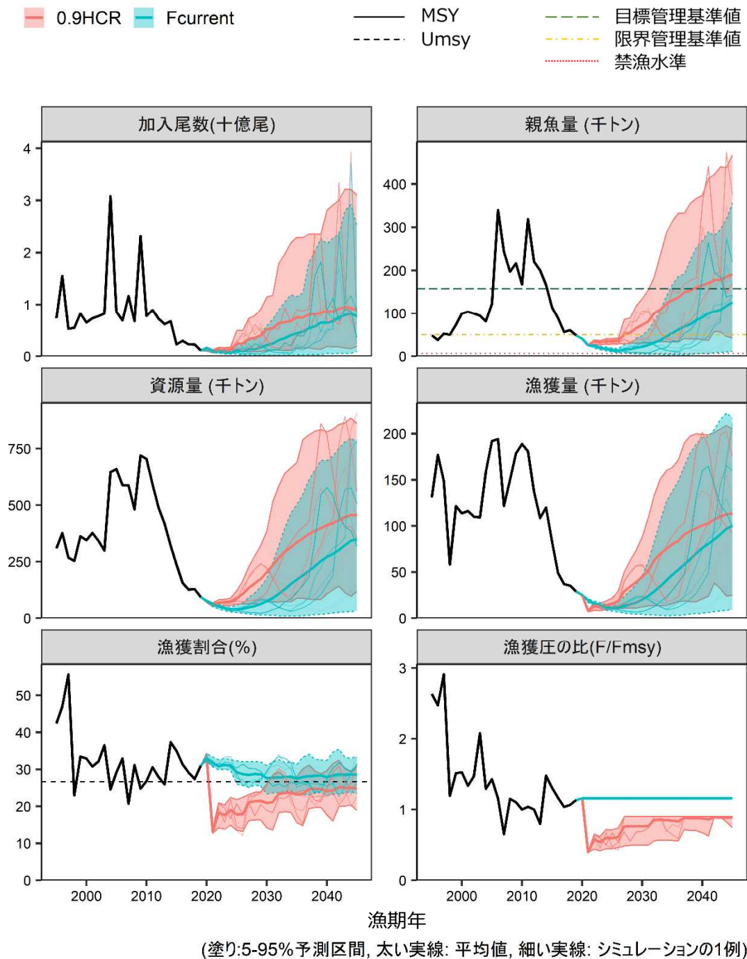
補足図 4-2. 管理基準値に基づく漁獲管理規則を用いた将来予測（赤色）と現状の漁獲圧で漁獲を続けた場合の将来予測（緑色）
