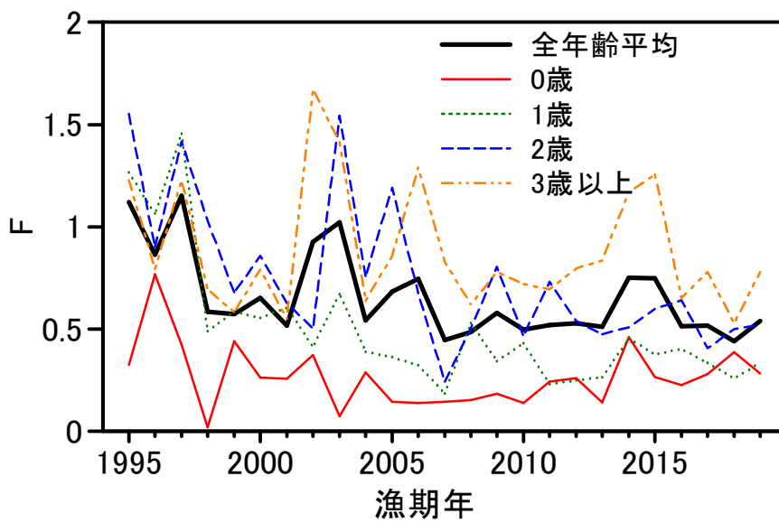
図 4-6. 年齢別漁獲係数 ( F ) の推移
