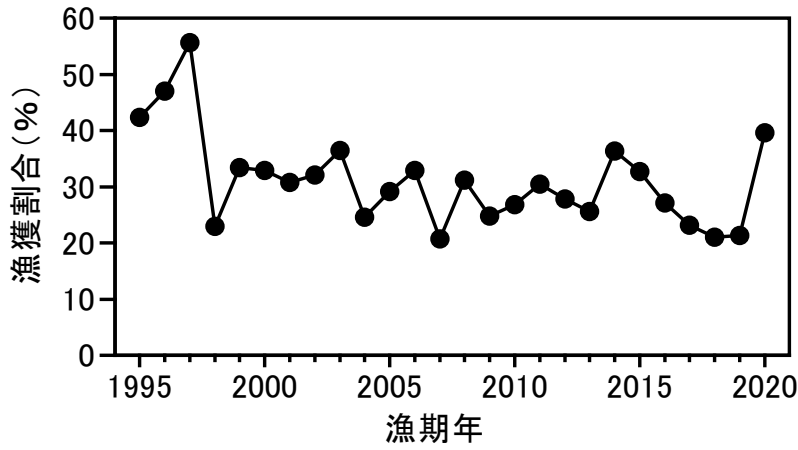
図 4-7. 漁獲割合の推移
