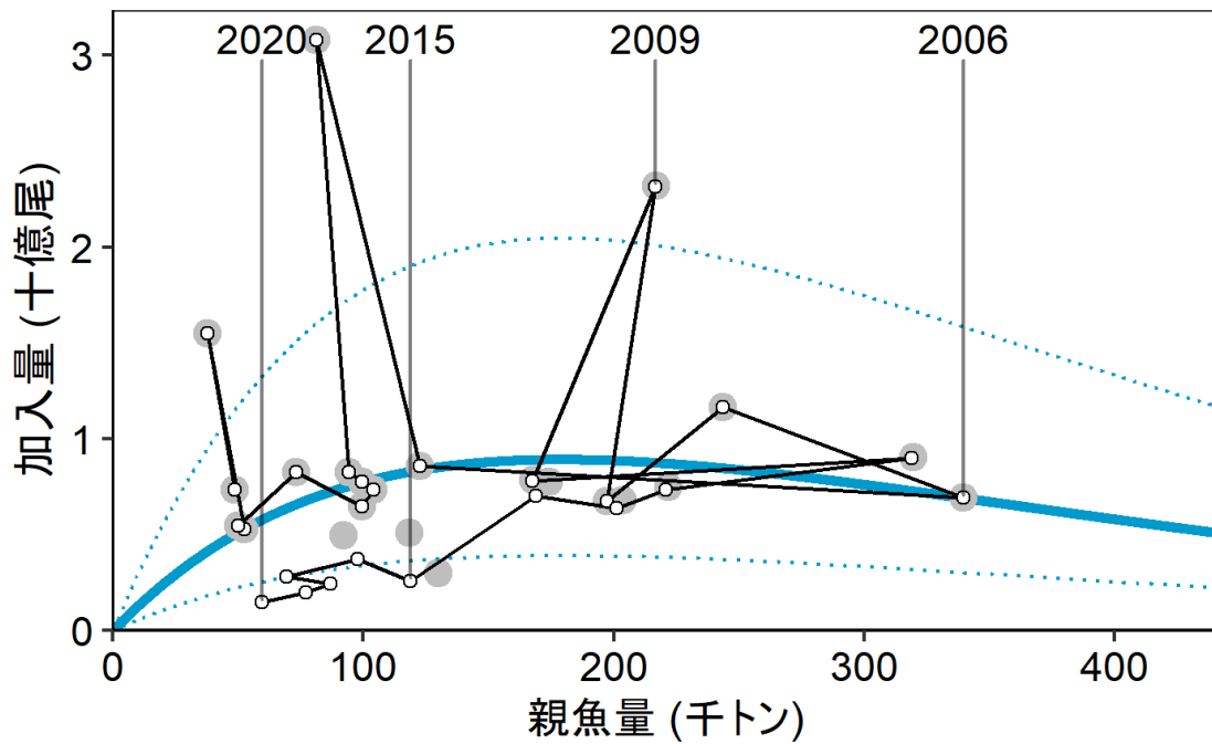
図 4-10. 親魚量と加入量の関係（再生産関係） 平成 31 年 4 月に開催された「管理基準値等に関する研究機関会議」（由上ほか 2019a）で提案された再生産関係式と再生産関係のプロット（灰色の丸印）。図中の再生産関係式（青線）の上下の点線は、仮定されている再生産関係において観察データの 90%が含まれると推定される範囲である。実線と白抜き丸印で示したのは今年度の資源評価で得られた再生産関係のプロット。
