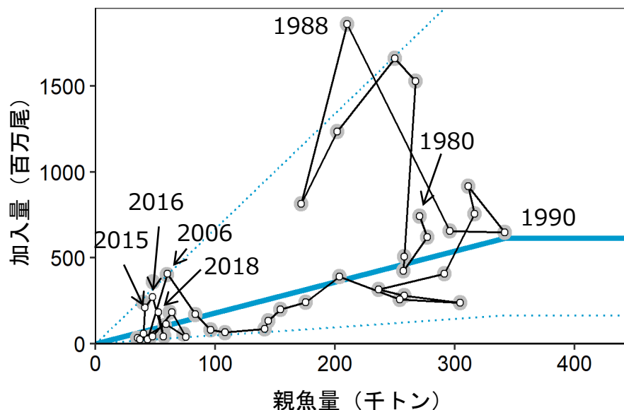
図4 再生産関係
