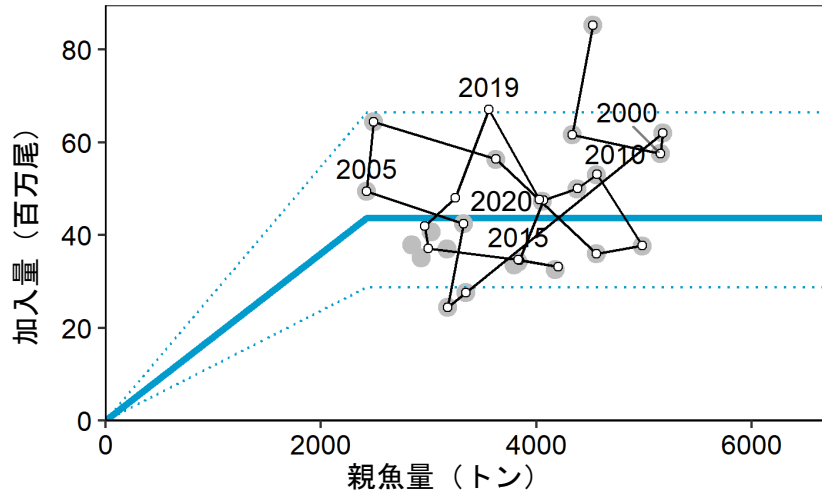
図4 再生産関係
