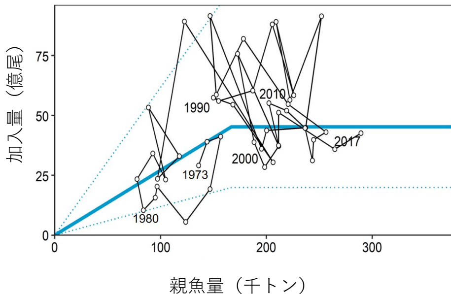
図4 再生産関係
