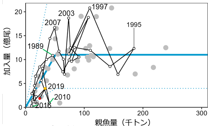
図4 再生産関係
