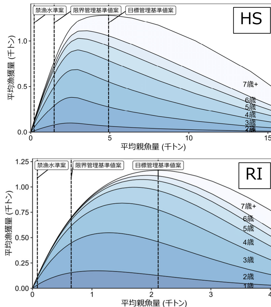
図15 HS型（上）とRI型（下）再生産関係による管理基準値案と禁漁水準案
