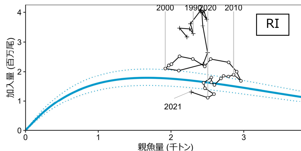
図13 リッカー（RI）再生産関係
