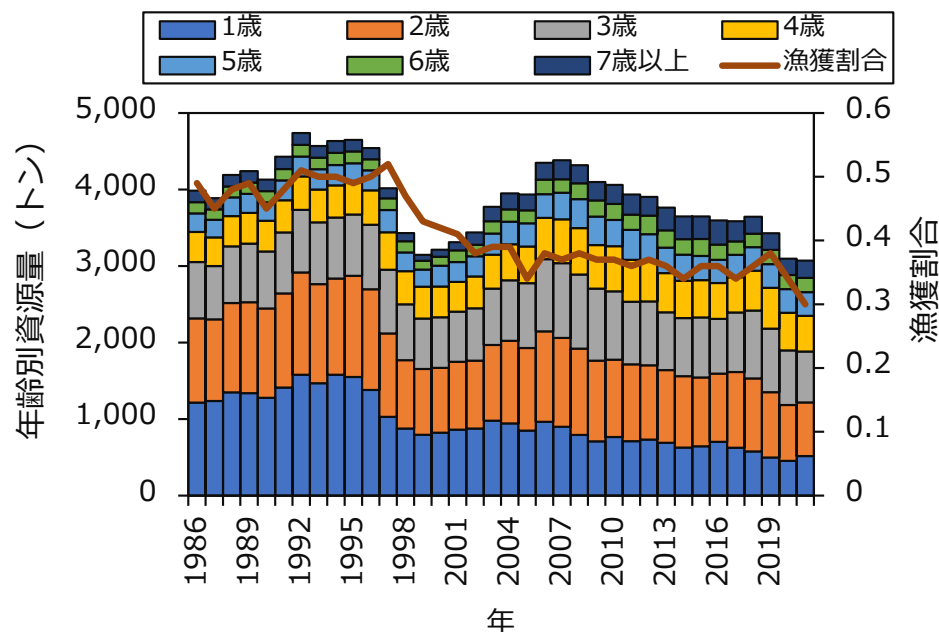
図4 年齢別資源量と漁獲割合の推移
