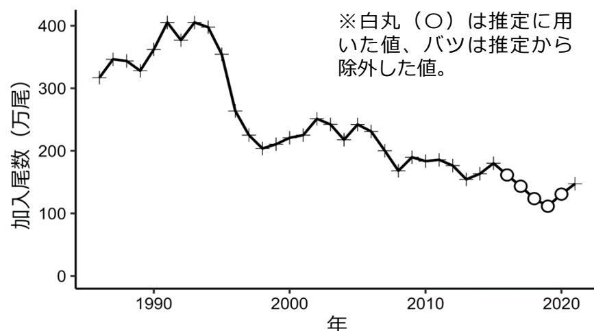
図6 天然由来の加入量の時系列
