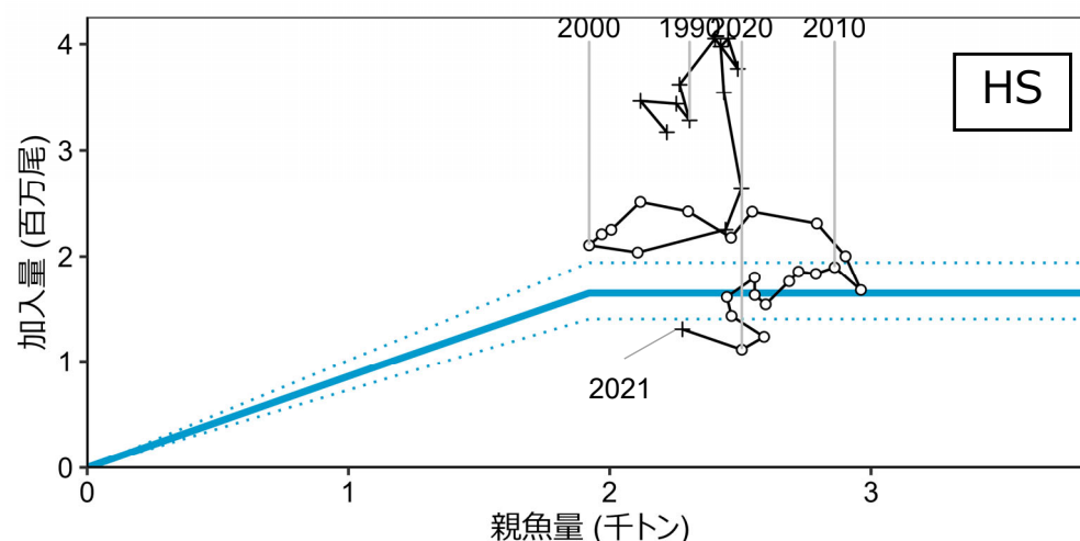
図12 ホッケー・スティック（HS）再生産関係
