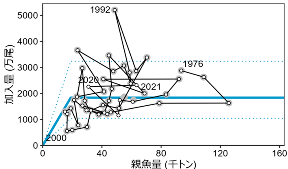
図6 再生産関係
