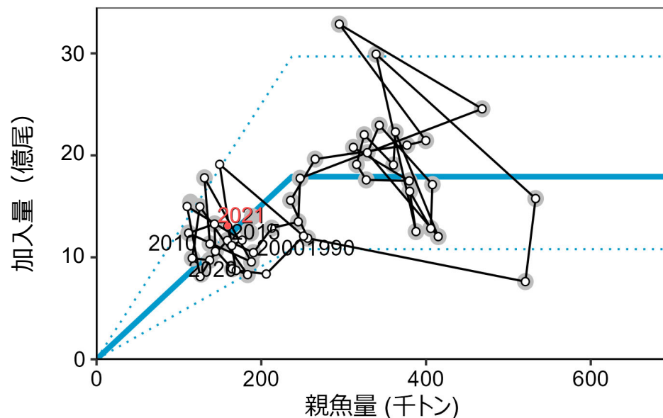
図6 再生産関係
