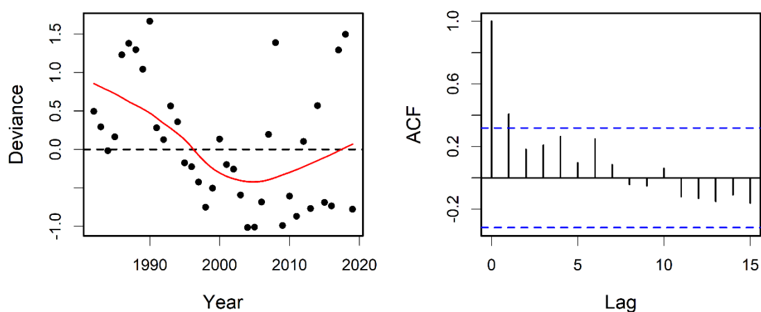
図 A-3. ホッケースティック型再生産関係における残差トレンドと自己相関プロット
