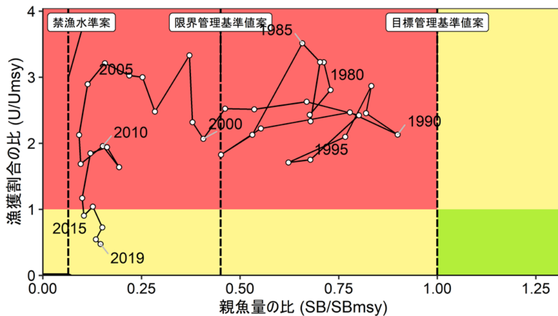
図 A-5. 更新された最大持続生産量に関わる管理基準値を基準にした神戸プロット
