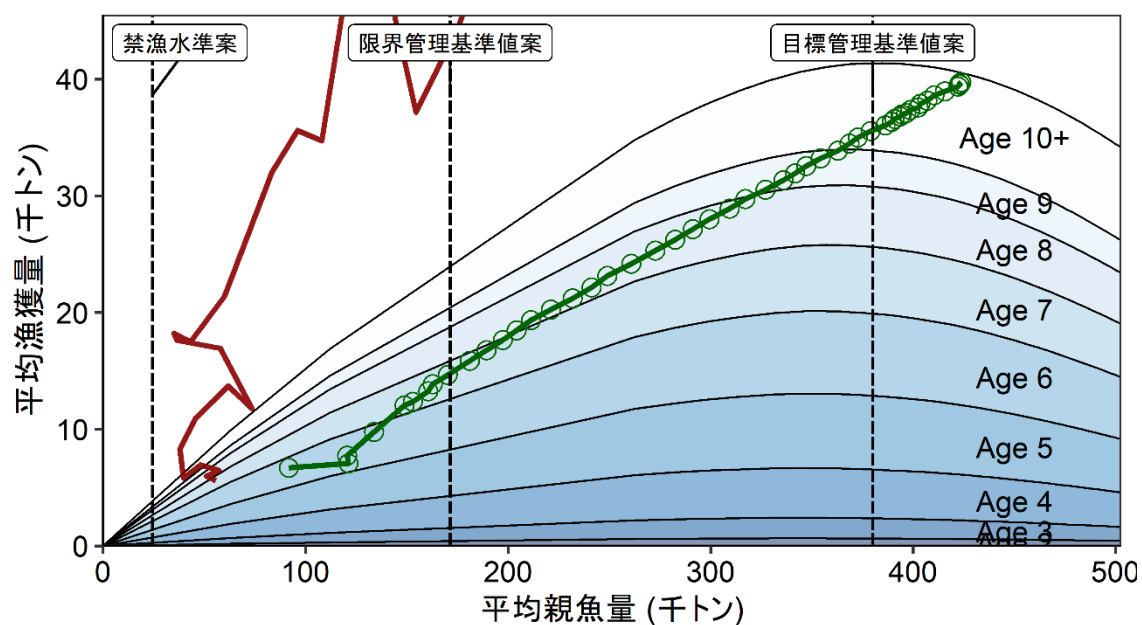
図 A-4. 管理基準値案と年齢別漁獲量曲線の関係
