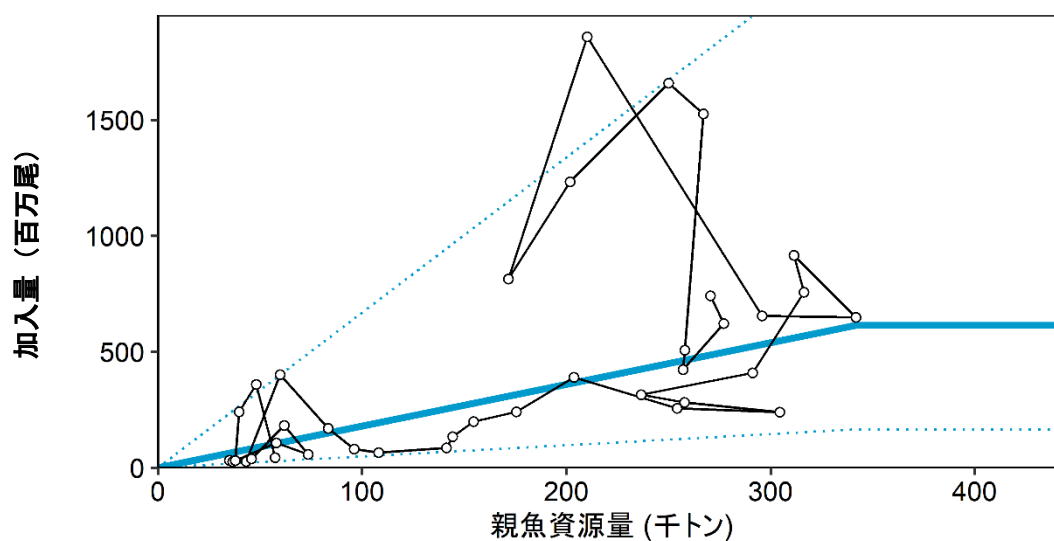
図 A-1. 更新した再生産関係式（親魚量と加入量の関係）
