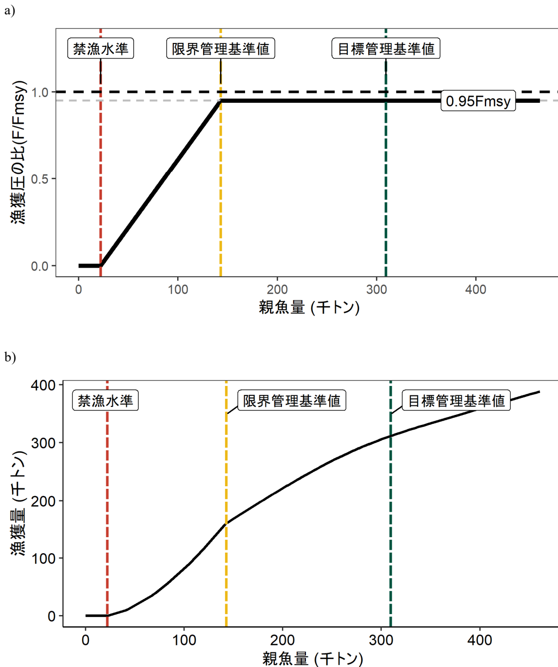
図 5-1. 漁獲管理規則（調整係数 \beta=0.95 の場合）。目標管理基準値 (SBtarget) はホッケ-スティック型再生産関係に基づき算出した SB_{msy} である。限界管理基準値 (SBlimit) および禁漁水準 (SBban) にそれぞれ標準値を用いている。黒破線： F_{msy} 、灰色破線： 0.95F_{msy} 、黒太線：HCR、赤破線：禁漁水準、黄色破線：限界管理基準値、緑色破線：目標管理基準値を示す。a) は縦軸を漁獲圧にした場合、b) は縦軸を漁獲量で表した場合である。b) については、漁獲する年の年齢組成によって漁獲量は若干異なるが、ここでは平衡状態における平均的な年齢組成の場合の漁獲量を示した。
