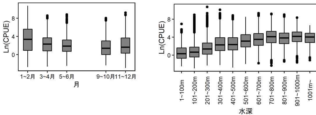
補足図 2-1. 月別（左）および水深帯別（右）の対数化した CPUE を示す箱ひげ図
