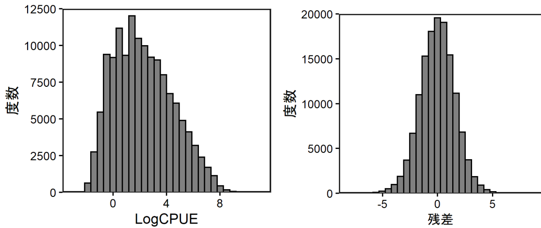
補足図 2-3. 対数化した日別船別 CPUE (左) とモデル予測値と実測値の残差 (右) のヒストグラム (1972~2021 年データ)
