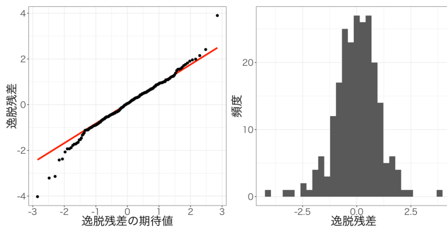
図 5. 各地区のモデルにおける QQ プロット (左) および残差の頻度分布 (右)
