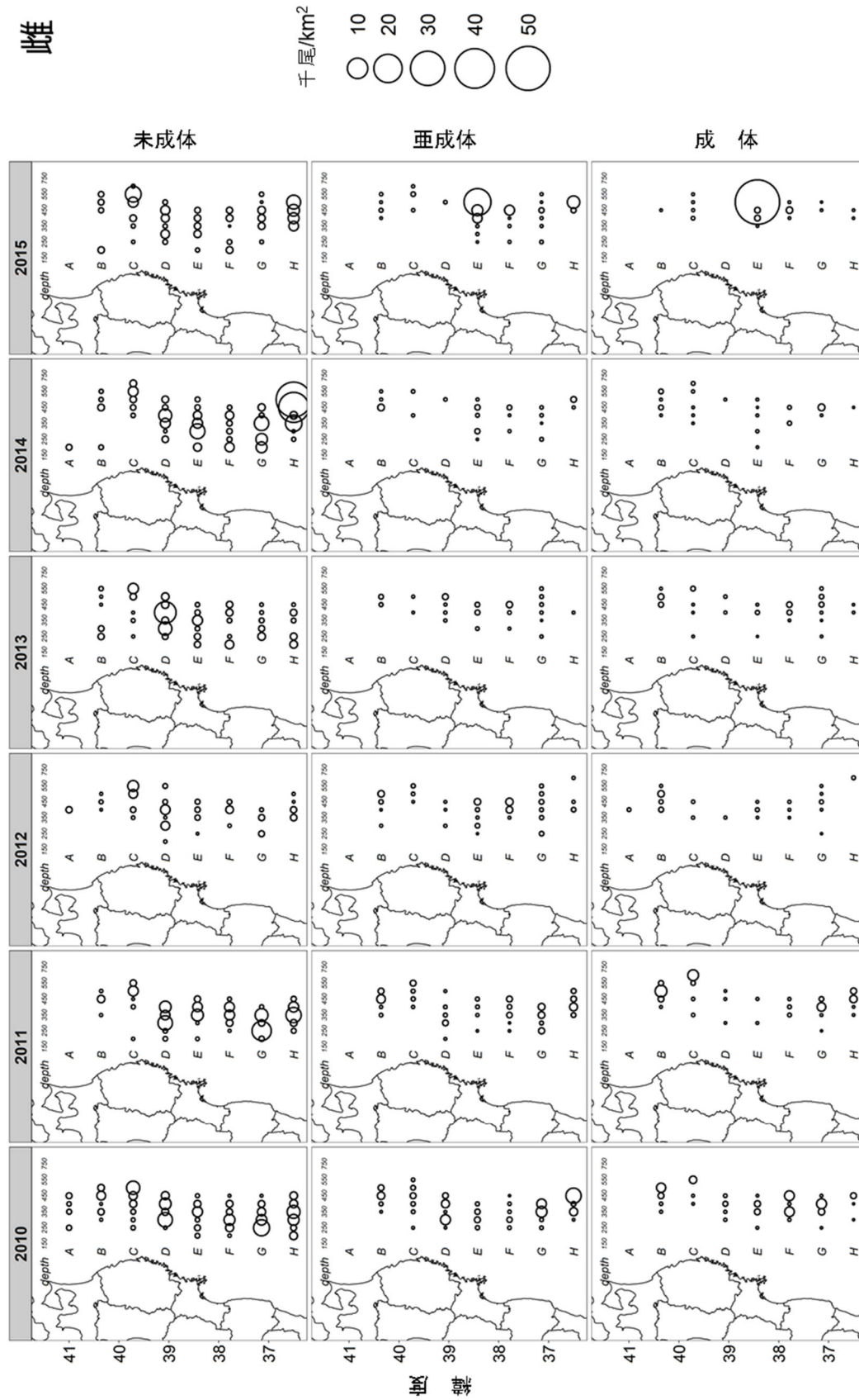
補足図 3-6. 2010～2015 年における雌の調査地点別の分布密度
