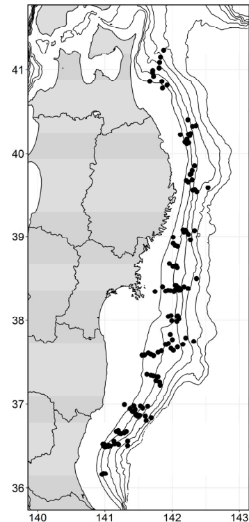
補足図 3-1. 2021 年の着底トロール調査点
