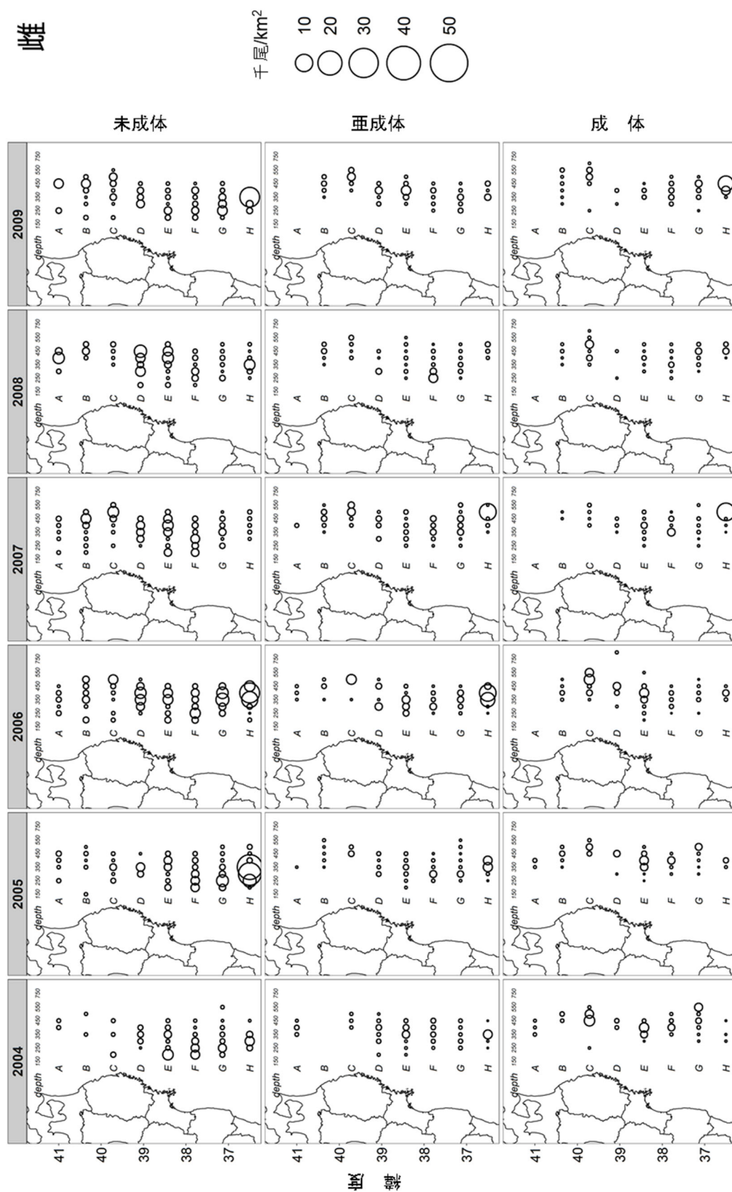
補足図 3-5. 2004～2009 年における雌の調査地点別の分布密度
