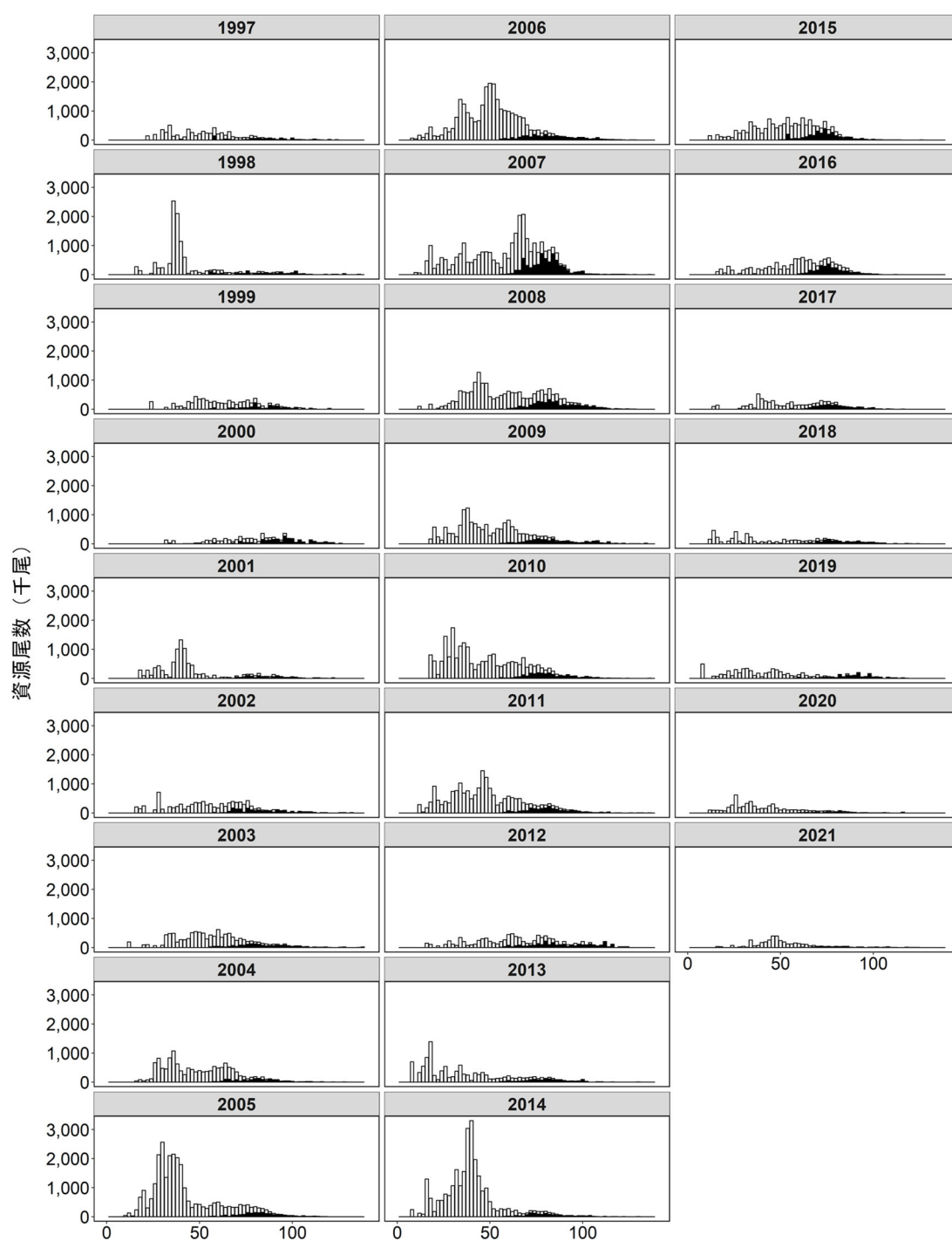
補足図 4-1. 雄の甲幅別現存尾数
