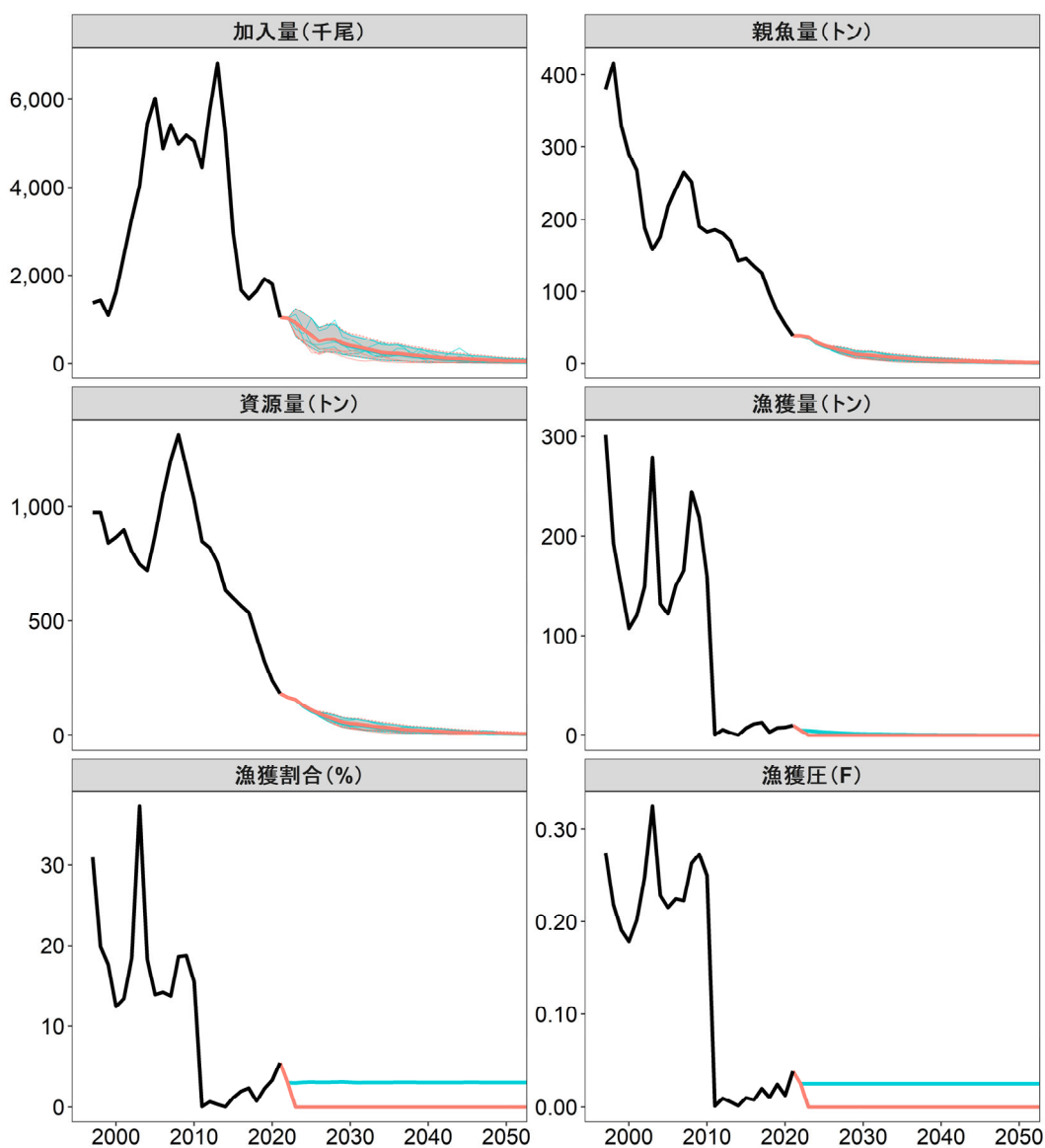
図 5-1. 現状の漁獲圧 (F2019-2021) で漁獲を続けた場合の将来予測 (緑) と、漁獲を 0 とした場合の将来予測 (赤)
