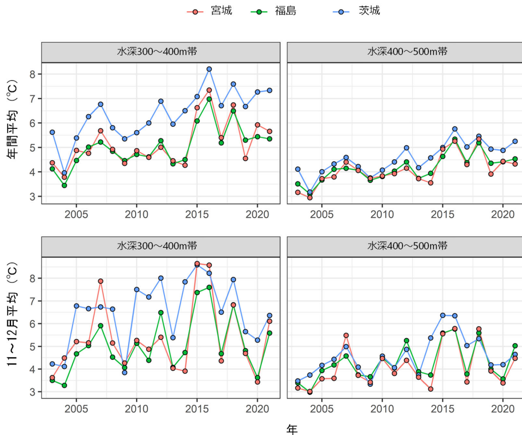
補足図 6-1. 東北沿岸各県別の底水温 (2006~2019 年)
