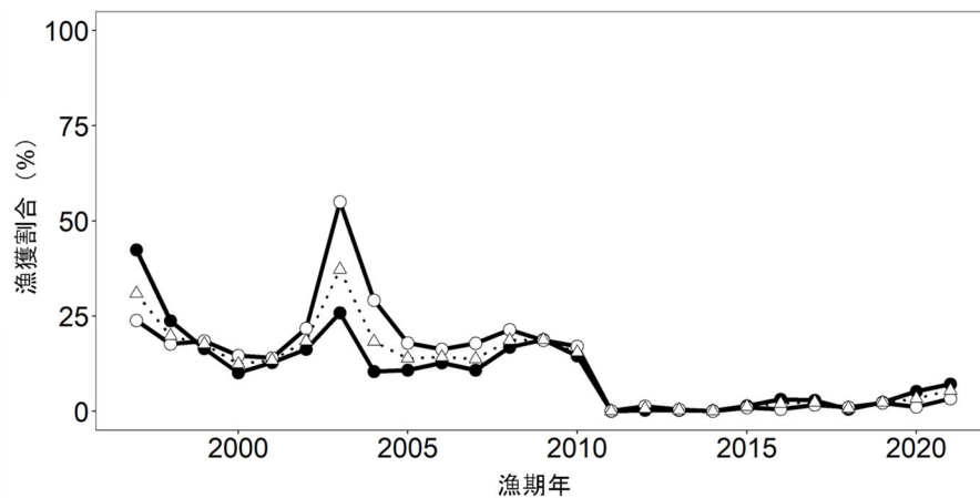
図 4-7. 漁獲割合 (雄：黒点、雌：白点、雌雄計：三角点) の推移
