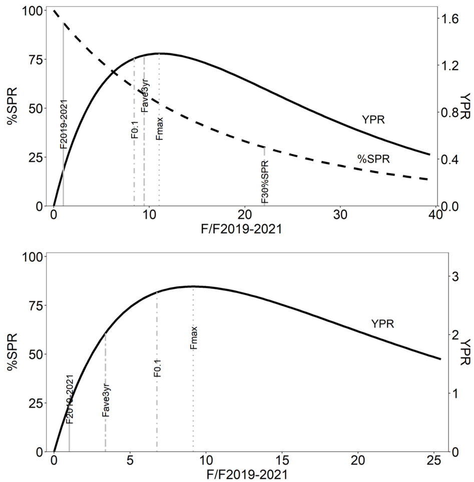
図 4-10. 雌雄別の F 値と YPR および %SPR の関係
