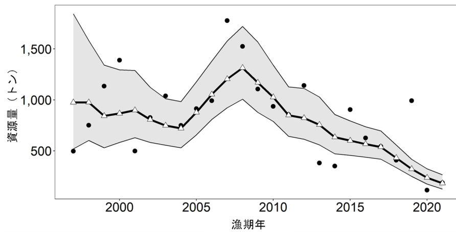
図 4-3. 漁獲対象資源量（三角点）、着底トロール調査による現存量（黒点）の推移 網掛けは推定値の 95%信頼区間を示す。
