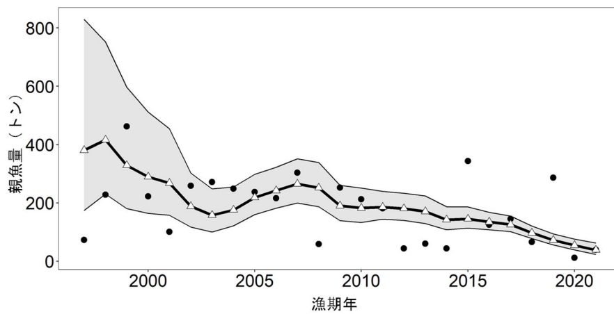
図 4-5. 親魚量 (SSB) の推移
