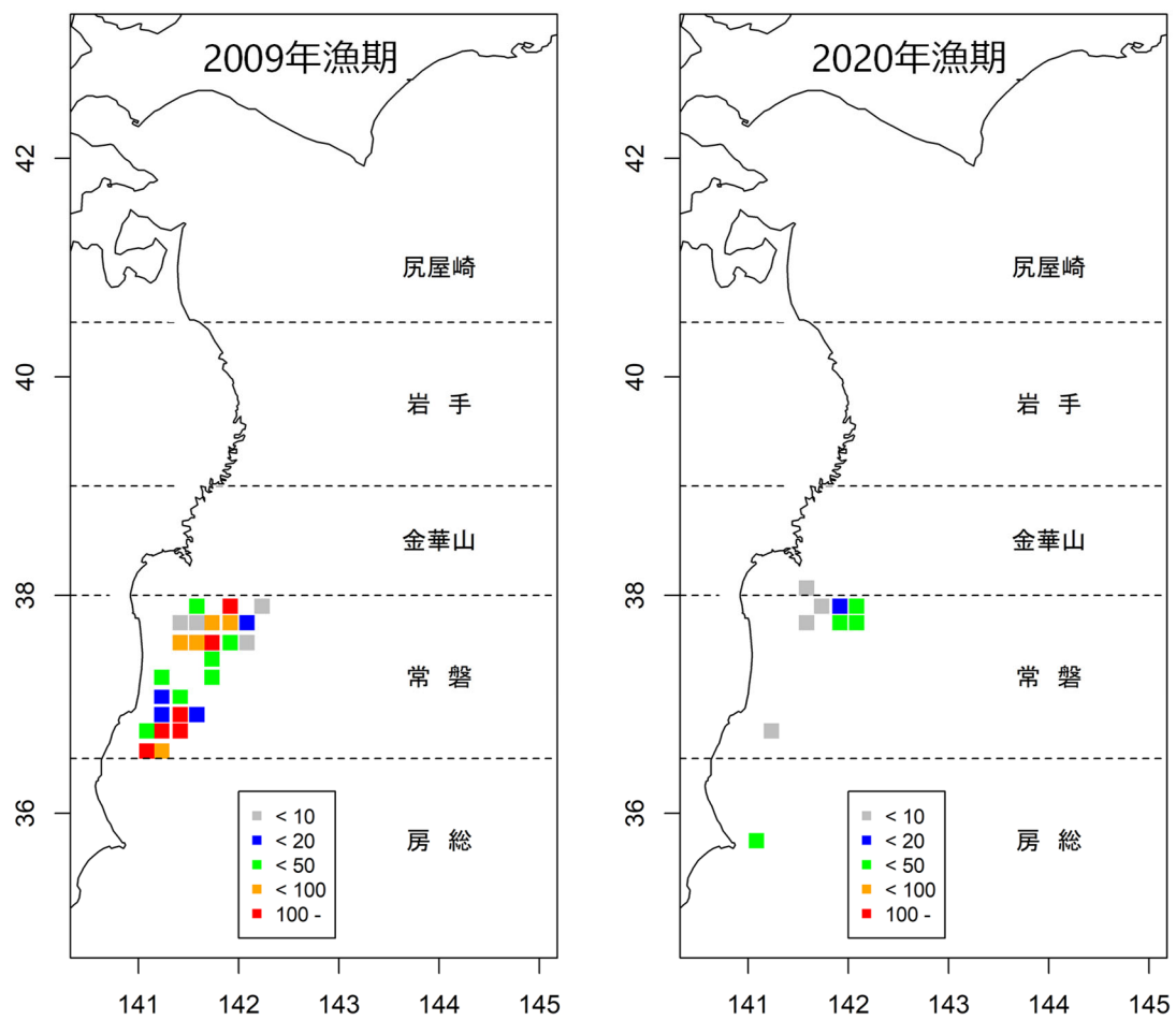
図 3-4. 震災前（2009 年漁期）と 2020 年漁期の漁獲努力量（有漁網数）の比較
