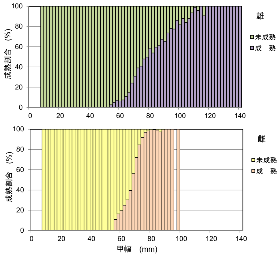
図 2-3. ズワイガニの甲幅別成熟割合 (1997～2021 年漁期)
