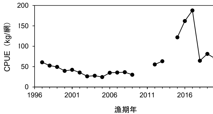
図 4-2. 福島県の沖底（トロール）によるズワイガニの CPUE
