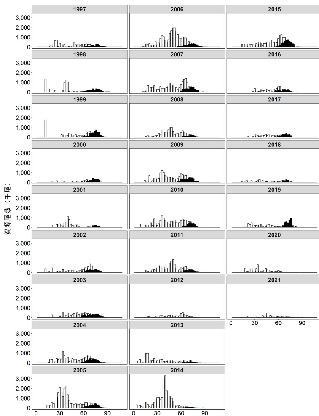
補足図 4-2. 雌の甲幅別現存尾数
