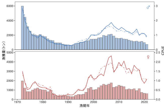
補足図 7-4. 雌雄別漁獲量（棒グラフ）、標準化 CPUE（実線）およびノミナル CPUE（点線） 標準化 CPUE およびノミナル CPUE はいずれもそれぞれの平均値で除して標準化した。
