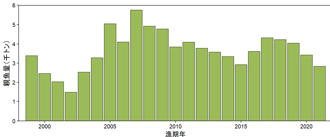
図 4-6. 親魚量の経年変化 本海域の親魚量は雌の漁期後資源量である。
