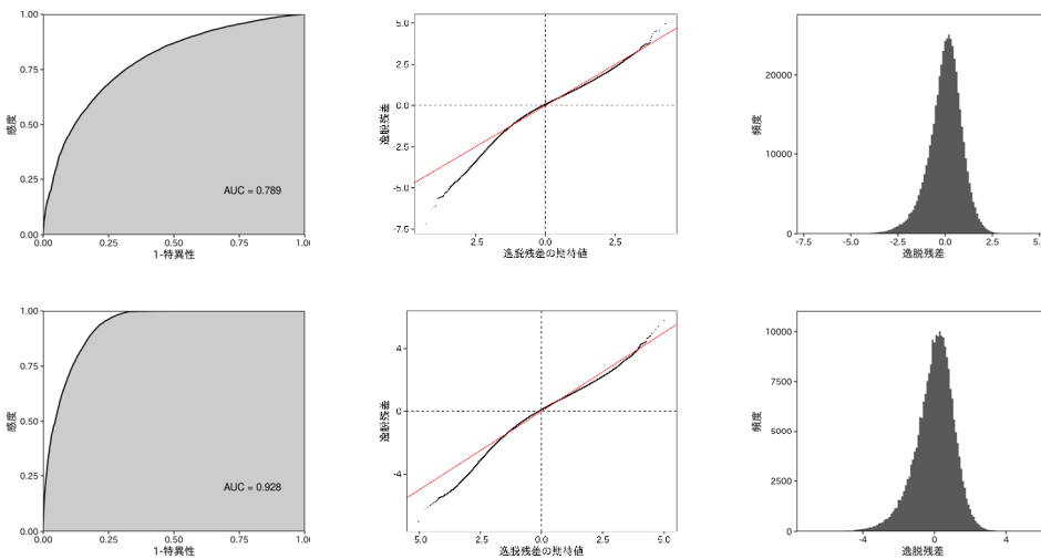
補足図 7-2. 雄（上段）および雌（下段）の有漁確率モデルに関する ROC 曲線（左）、有漁 CPUE モデルの QQ プロット（中）および逸脱度残差のヒストグラム（右）
