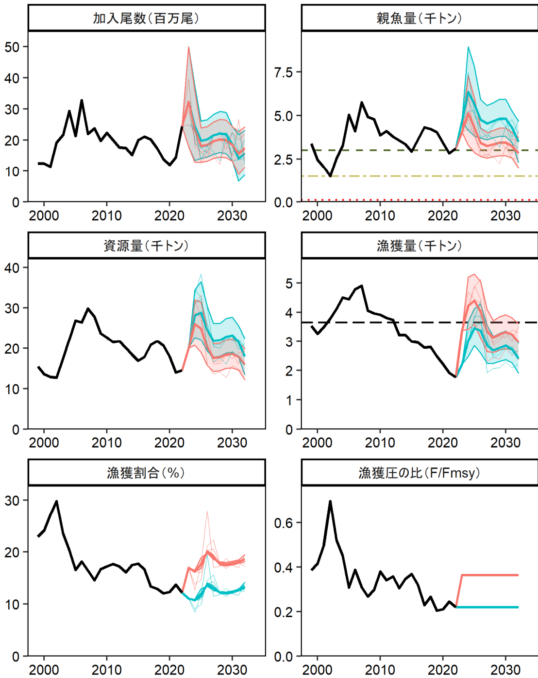
図 5-2. 漁獲シナリオで定められた管理基準値に基づく漁獲管理規則を用いた将来予測（赤色）と現状の漁獲圧で漁獲を続けた場合の将来予測（青色） 実線は平均値、網掛けはシミュレーション結果の90%が含まれる90%予測区間、細線は3通りの将来予測の例示である。親魚量の図の緑破線は目標管理基準値、黄鎖線は限界管理基準値、赤点線は禁漁水準を示す。2022年の漁獲量は予測される資源量とF2019-2021により仮定した。調整係数 \beta には0.8を用いた。
