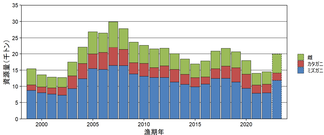
図 4-5. トロール調査結果に基づくコホート解析により推定された漁期開始時点の資源量 ミズガニとカタガニは 12 歳と 13 歳の合計を、雌は 11 歳をそれぞれ示す。 2023 年は、2022 年の 10 歳以上の齢期別資源尾数等から前進計算により求めた予測値。
