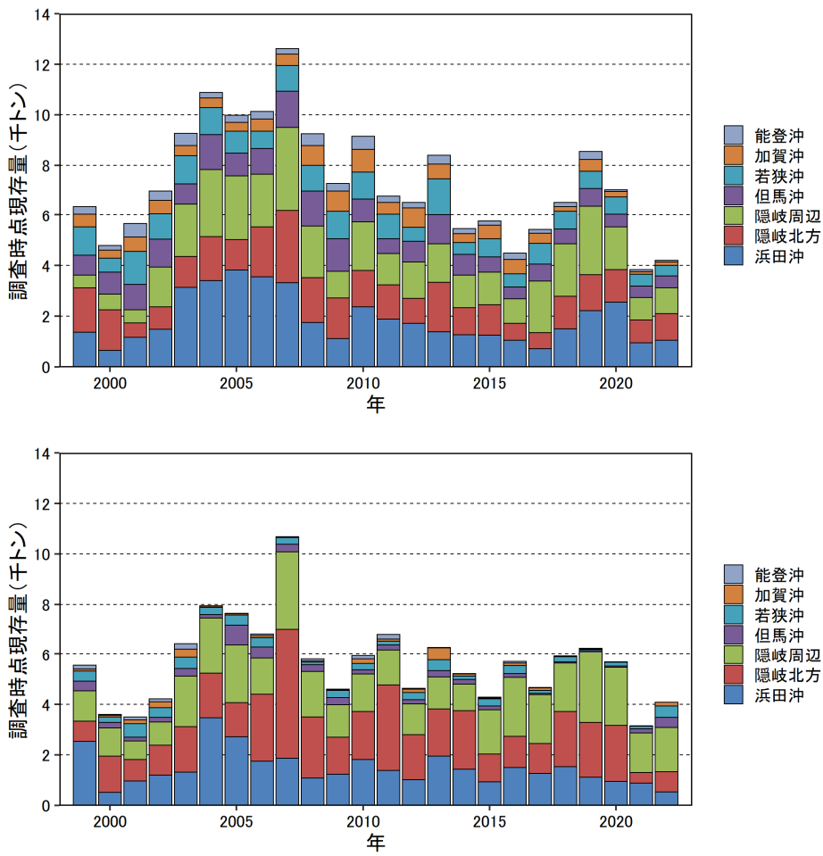
補足図 4-3. トロール調査から推定された海域別現存量 雄（上図）は甲幅 90 mm 以上、雌（下図）は 11 歳の現存量を示す。
