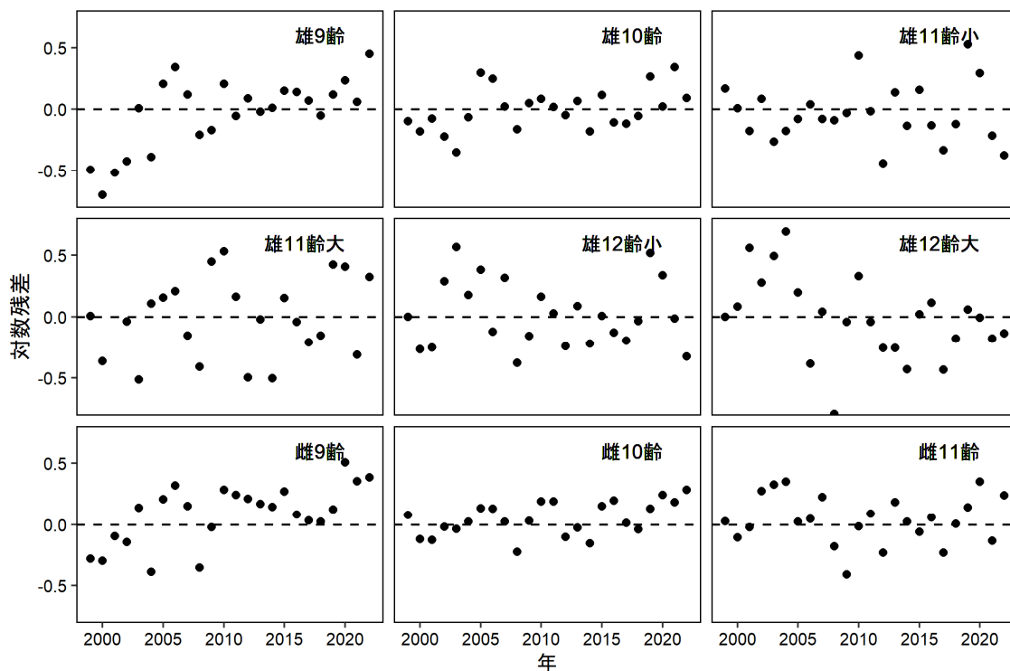
補足図 2-3. トロール調査による年別齢別現存尾数の観測値（対数）に対する推定値（対数）の残差点線は0を、縦軸は残差を、「小」は鉈脚小（未成熟・最終脱皮前）を、「大」は鉈脚大（成熟・最終脱皮後）を、それぞれ示す。
