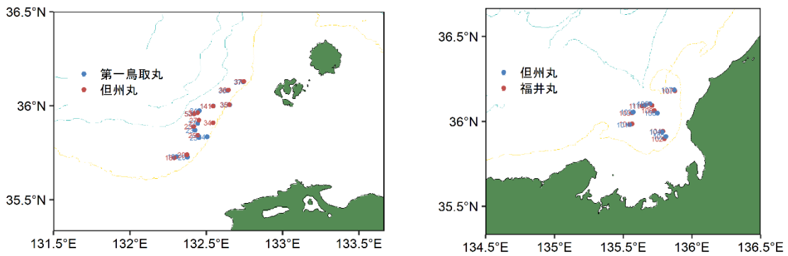
補足図 4-4. 隠岐西方（左図）および若狭沖（右図）での並行操業における調査点
