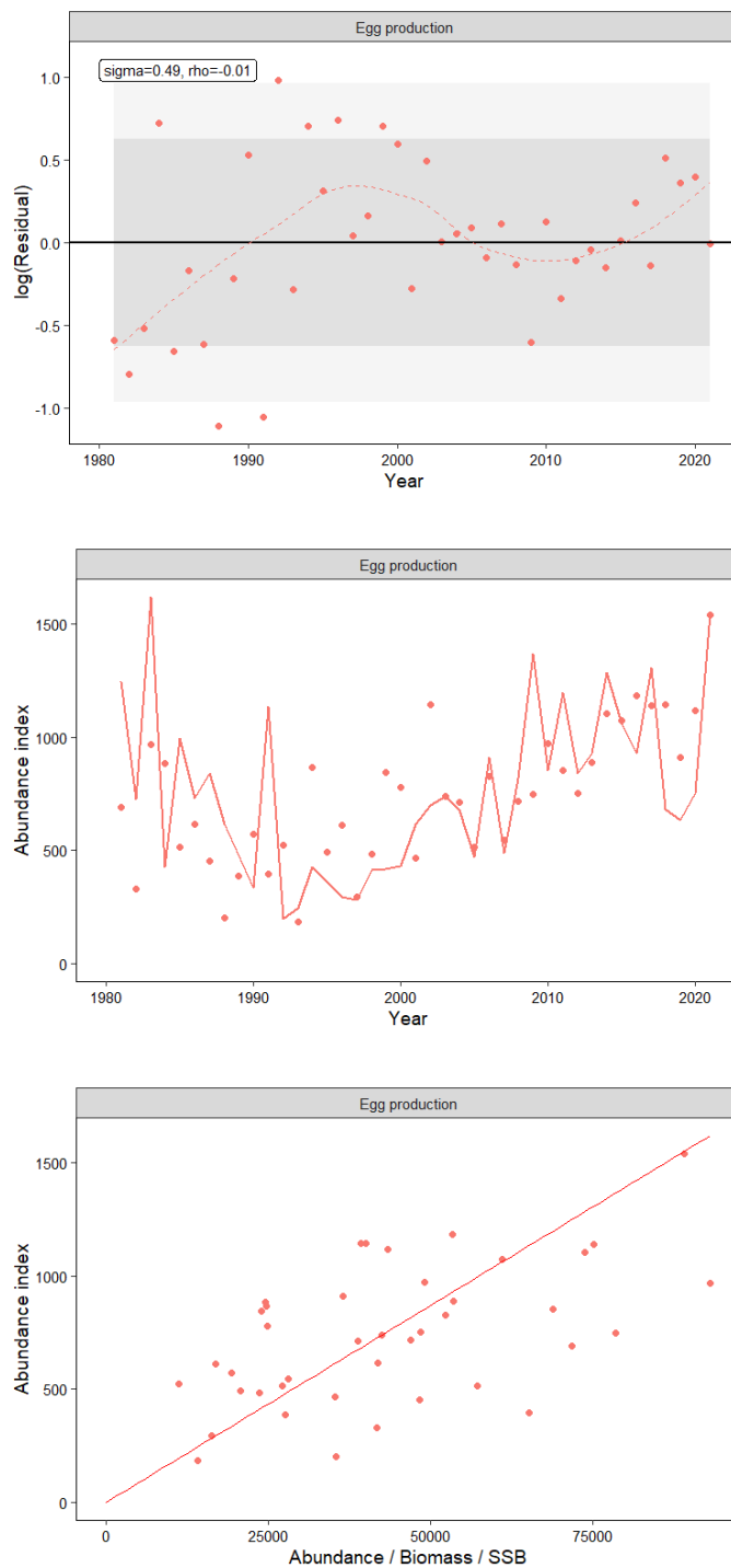
補足図 2-2. 資源量指標値と予測値の関係
