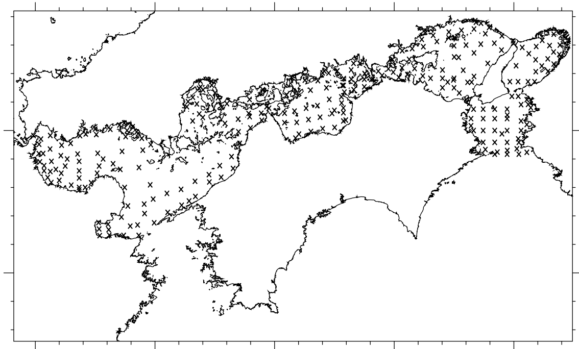
補足図 2-3. 瀬戸内海の卵稚仔調査における調査点（×）の配置図
