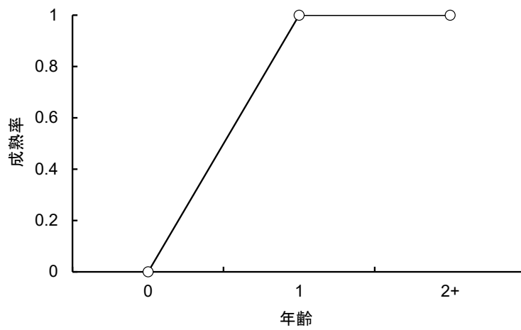
図 3. 年齢と成熟率
