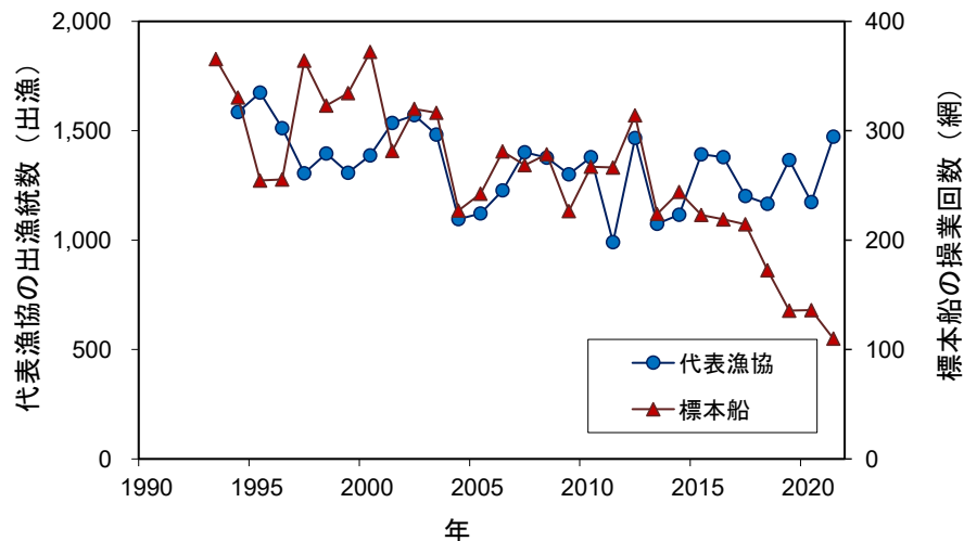
補足図 4-2. シラス漁業における努力量の推移
