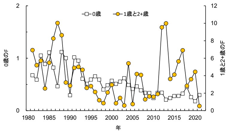
図 9. カタクチイワシの F の推移
