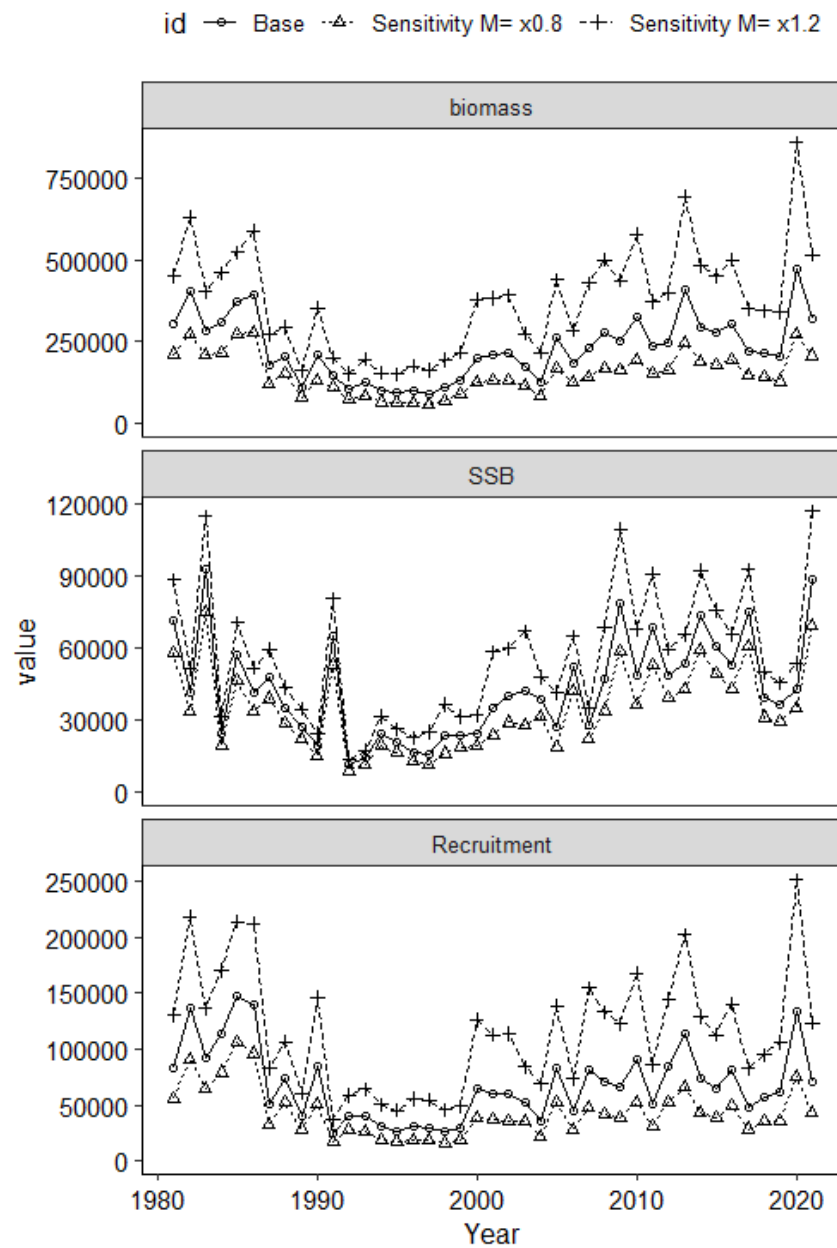
図 12. M の感度解析結果
