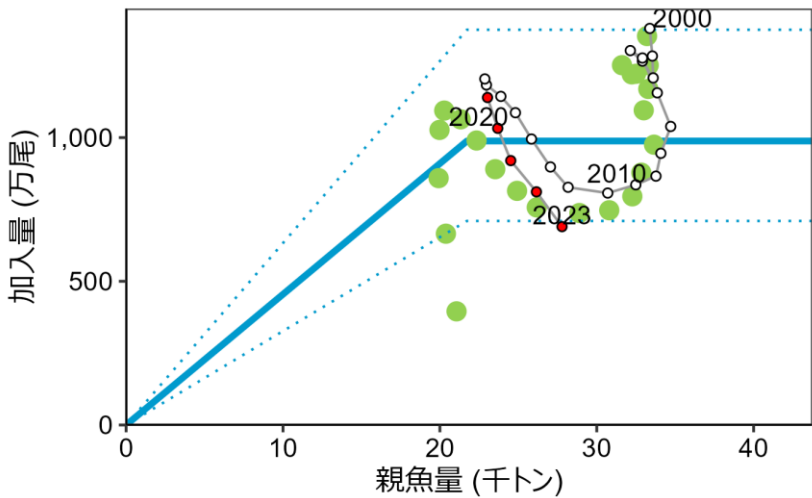
図7 再生産関係
