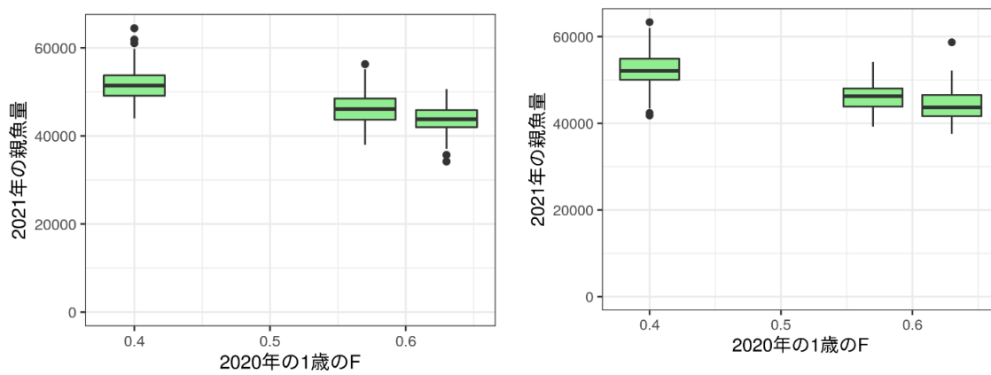
補足図 3-4. 2021 年の親魚量（トン）と 2020 年の 1 歳への F との関係。左：バックワード・リサンプリング。右：対数正規分布。
