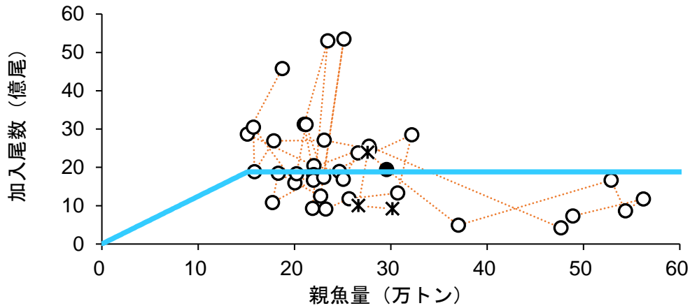
図 4-13. 親魚量と加入量の関係（再生産関係） 青線は平成 31 年 4 月に開催された「管理基準値等に関する研究機関会議」（境ほか 2019）で適用された再生産関係式。 *の加入量は調査からの推算値。 今回の資源評価で新たに推定された 2016 年級群を●で示す。
