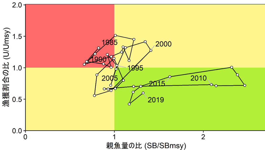
補足図 10-6. 更新された最大持続生産量に関する管理基準値を基準にした神戸プロット
