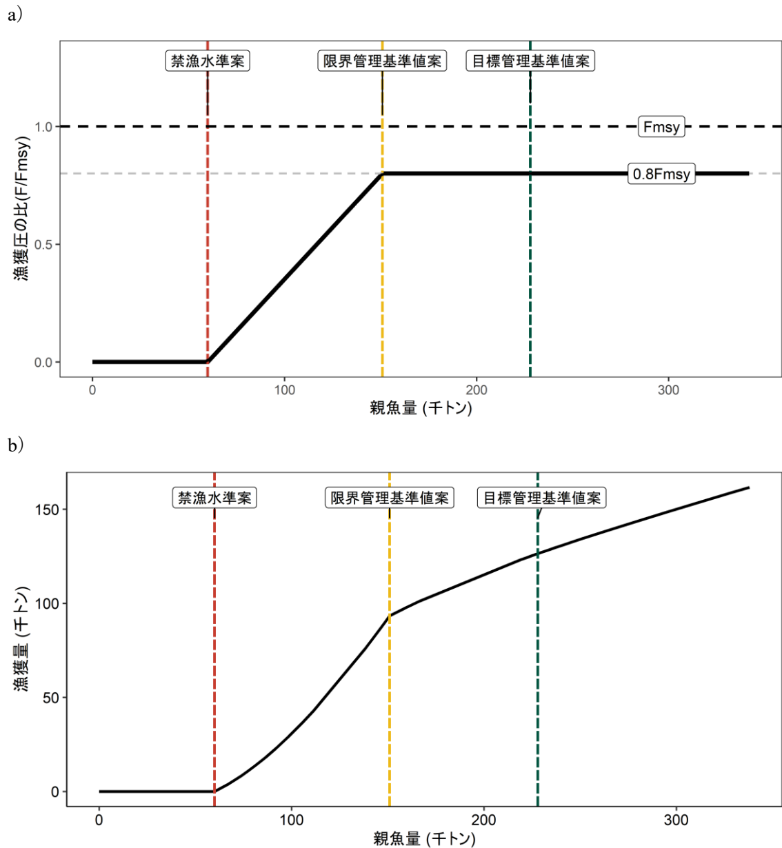
補足図 10-7. 漁獲管理規則案 ( \beta を 0.8 とした場合のものを示す)
