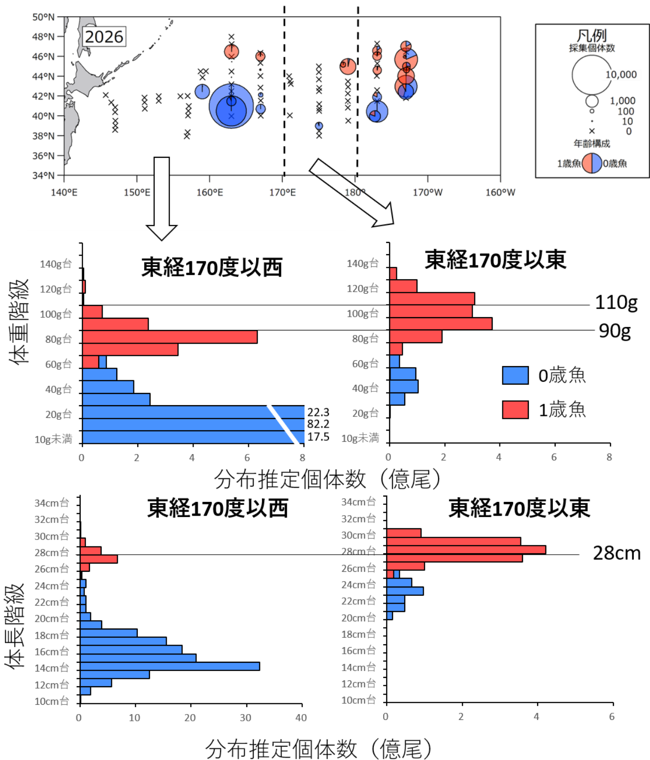
図 6. サンマ資源量直接推定調査結果をもとに推定された 1 区と 2 区（180 度以西）に分布していたサンマの海区別体重・体長組成。
