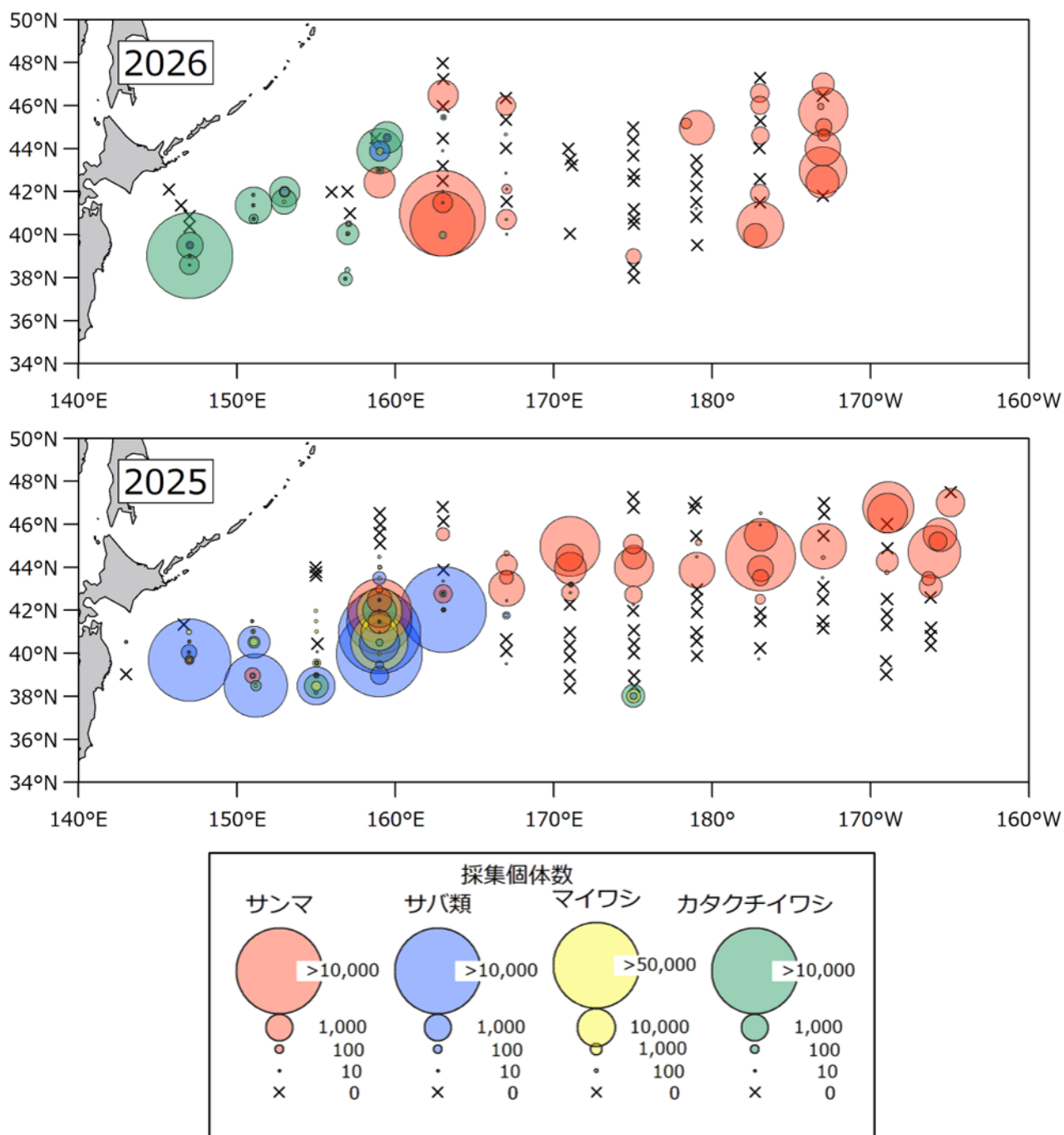
図7. サンマ資源量直接推定調査で採集されたサンマ（赤）、さば類（マサバおよびゴマサバ；青）、マイワシ（黄）、およびカタクチワシ（緑）の採集個体数。4 種とも採集されなかった調査点は×で示した。
