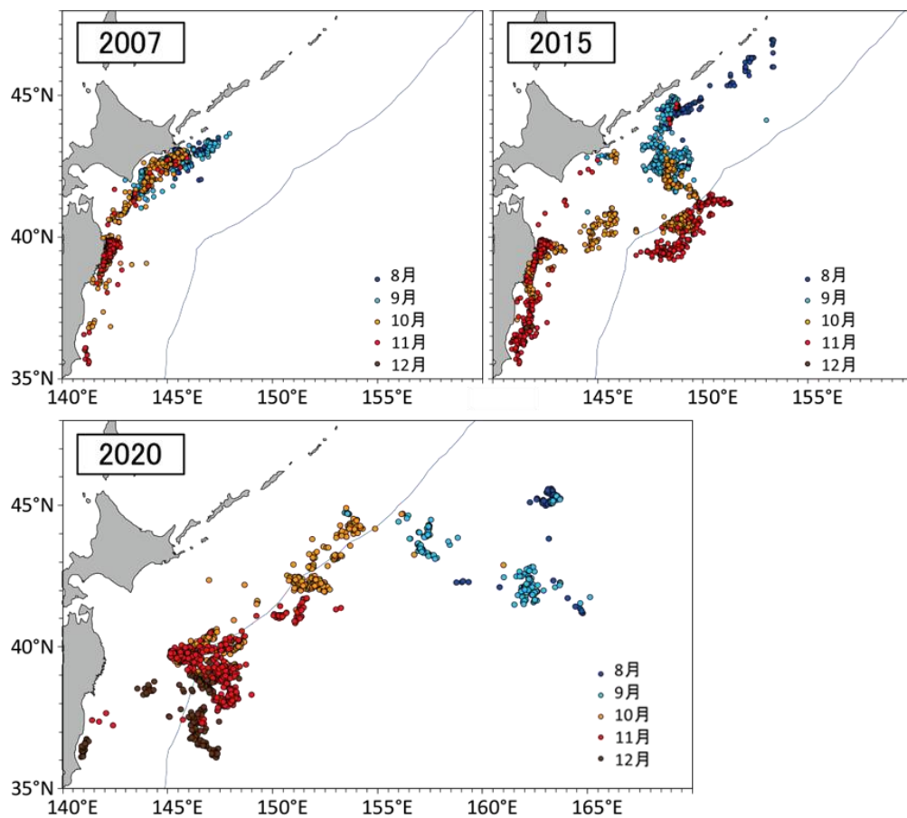
補足図 1-2. 月別のサンマの漁場。海洋環境や 6 月～7 月のサンマの分布の変化に伴い、近年漁場が沖合に移動している。
