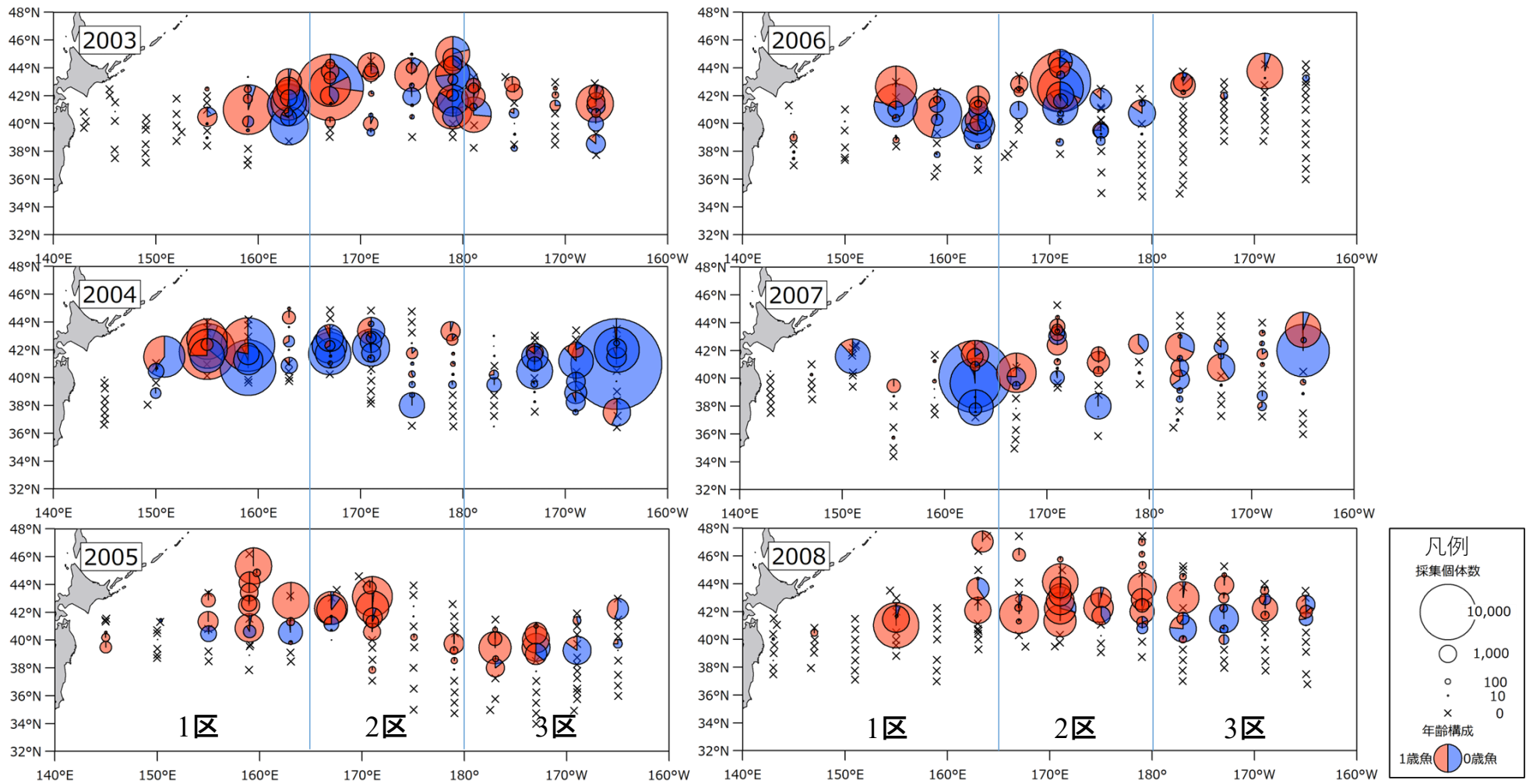
補足図 2-1. サンマ資源量直接推定調査におけるサンマの分布状況（2003 年～2008 年）。円の面積は調査 1 曳網あたりの採集個体数を示す。●は 0 歳魚、●は 1 歳魚の割合を示す。
