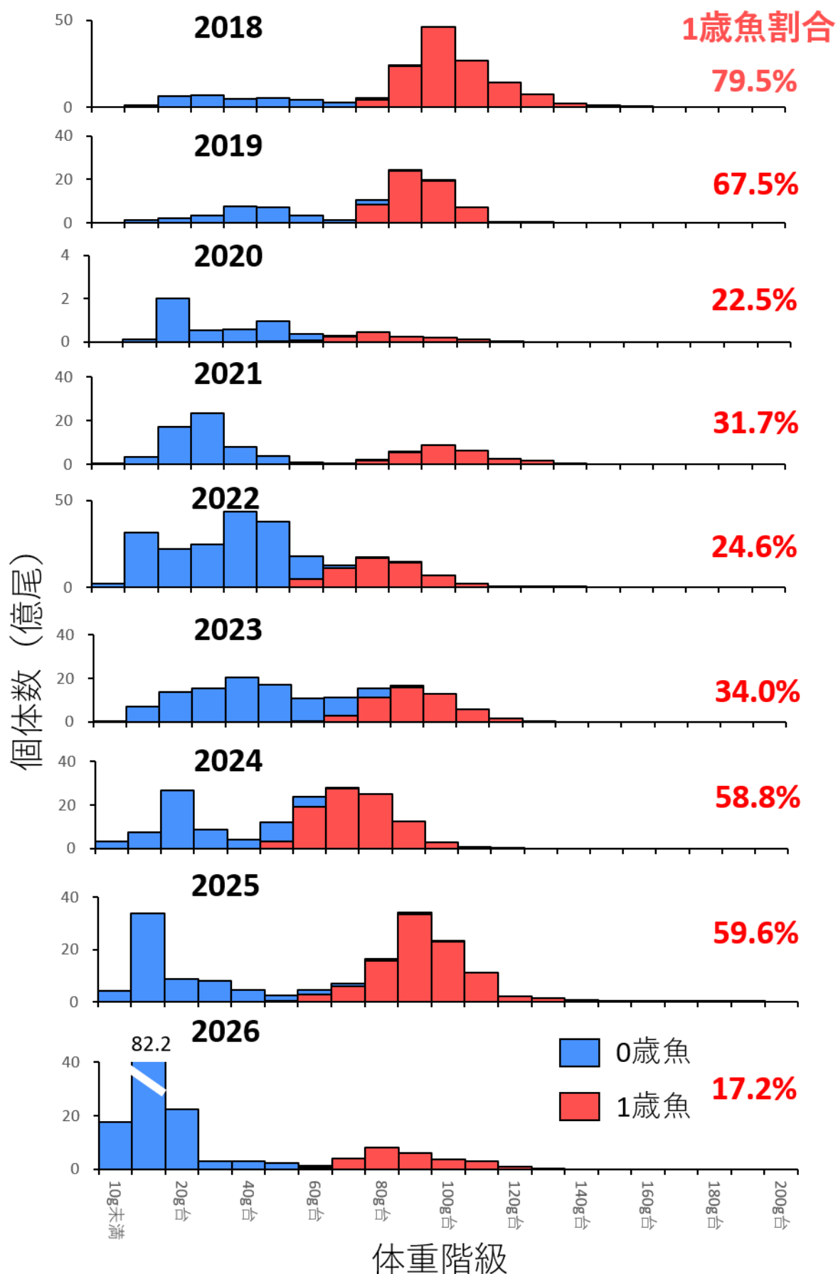
図 5. サンマ資源量直接推定調査結果をもとに推定された 1 区と 2 区（180 度以西）に分布していたサンマの体重組成の経年変化。年別の推定分布個体数のうちの 1 歳魚の割合を赤字で示した。
