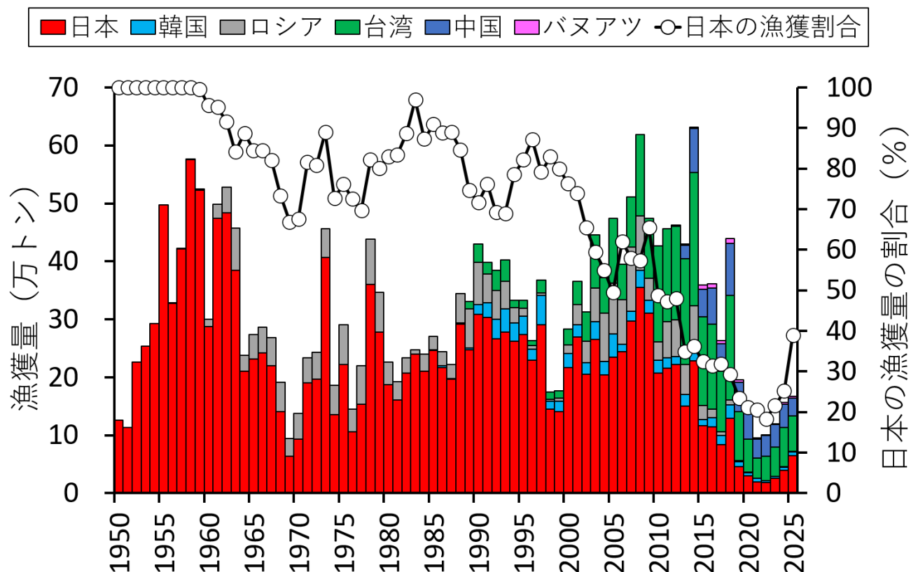
補足図 1-3. サンマ漁獲量の推移（1950 年～2025 年）と日本の漁獲割合。日本の漁獲量は海面漁業生産統計調査
