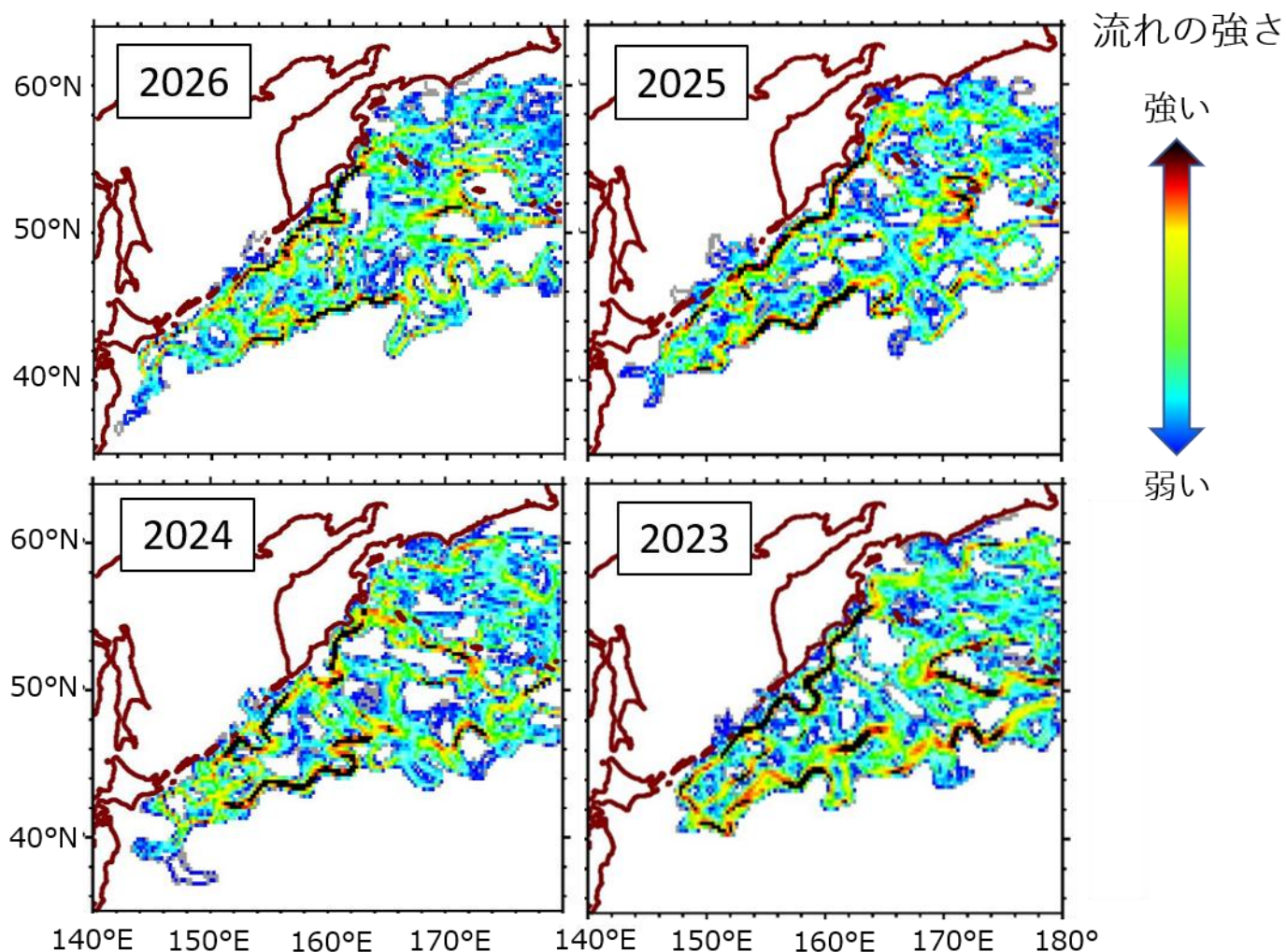
図 10. 人工衛星による海面高度データに基づいた 6 月の西部亜寒帯循環の流路の推移。西部亜寒帯循環は北西太平洋亜寒帯全域の海流の循環であるが、親潮はその南西端にあたる。人工衛星の海面高度計によって得られるデータから、この海流の強さと流路を推定することができる。図の黒い線は流れの強い本流を表しているが、2000 年代からの西部亜寒帯循環の弱まりに伴い、近年はこの本流が日本近海に達しなくなる傾向がみられる。2023 年は千島列島沿いに南西に流れた親潮の本流が道東近海に達することなく南東に反転し、北緯 40 度付近まで達した。一方、2024 年、2025 年は釧路沖や北緯 39 度付近まで親潮が広がっていた。2026 年も 2025 年と同等の張り出しが認められる。分析方法は、Kuroda et al. (2021) 参照。
