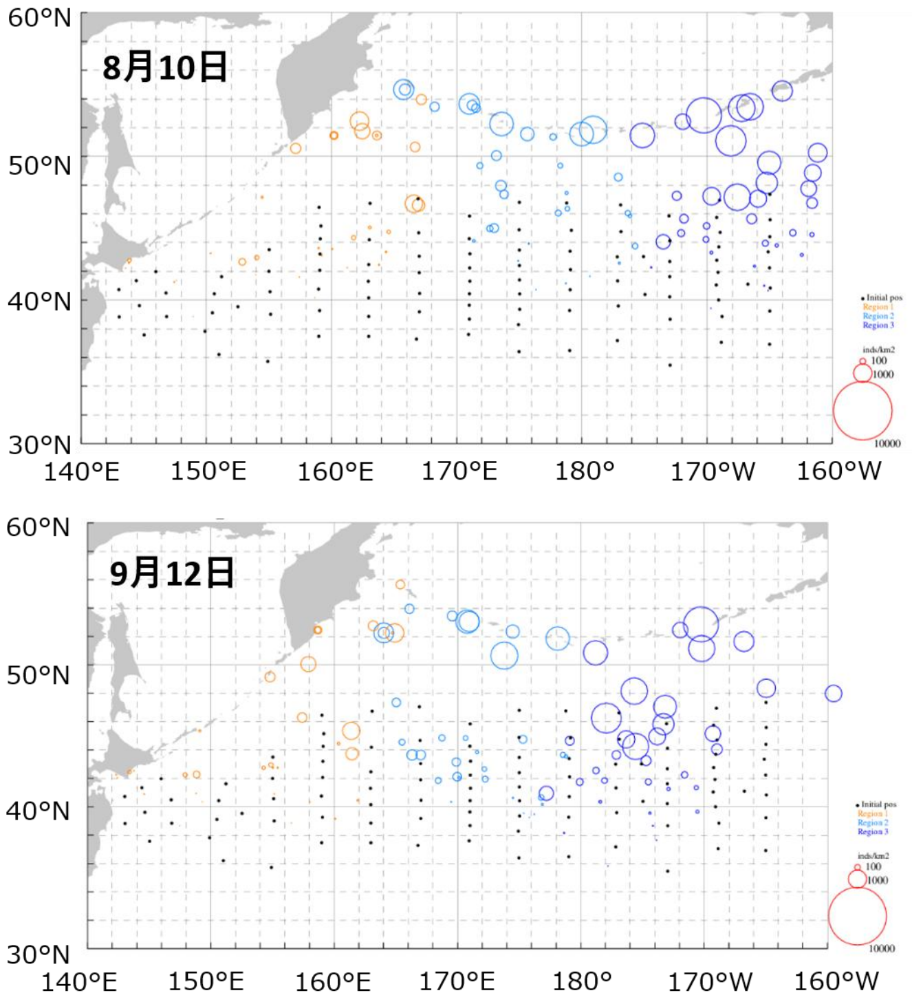
図 8. FRA-ROMSIIによる水温・海流予測とサンマの回遊特性を組み合わせた回遊モデルによる来遊予測。5月～7月に行われたサンマ資源量直接推定調査結果を用いて推定されたサンマの分布をもとに、9月12日までにサンマが到達する海域を回遊モデルで推定した。モデルは、サンマは8月26日まで等温線の北上とともに北に回遊し、その後は(0.7m/s【2.5BL/s, BL=体長】)で10日ごとに約0.3℃ずつ高水温帯を指向しつつ西側に回遊するように設定した。上の図は8月10日の、下の図は9月12日の予測位置を示す。丸の大きさは回遊の始点(調査時)の推定分布個体数を、色は回遊の始点の経度区分を示す(オレンジ:1区(東経165度以西)、水色:2区(東経165度～180度)、青色:3区(180度以東))。詳しくはTakehi et al. (2022)参照。
