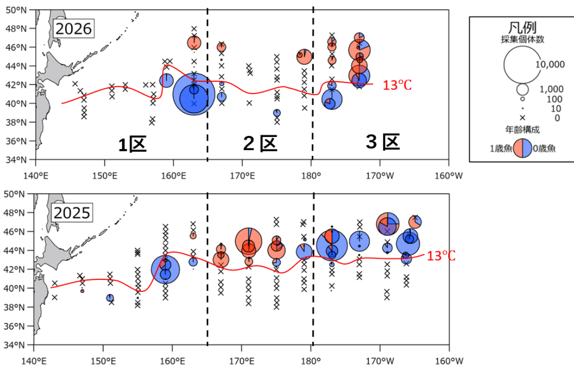
図2. 2026年および2025年におけるサンマ資源量直接推定調査の調査範囲と採集個体数。分布量の推定は、調査範囲を1区（東経165度以西）、2区（東経165度～180度）および3区（180度以東）の3海区に分けて行っている。
