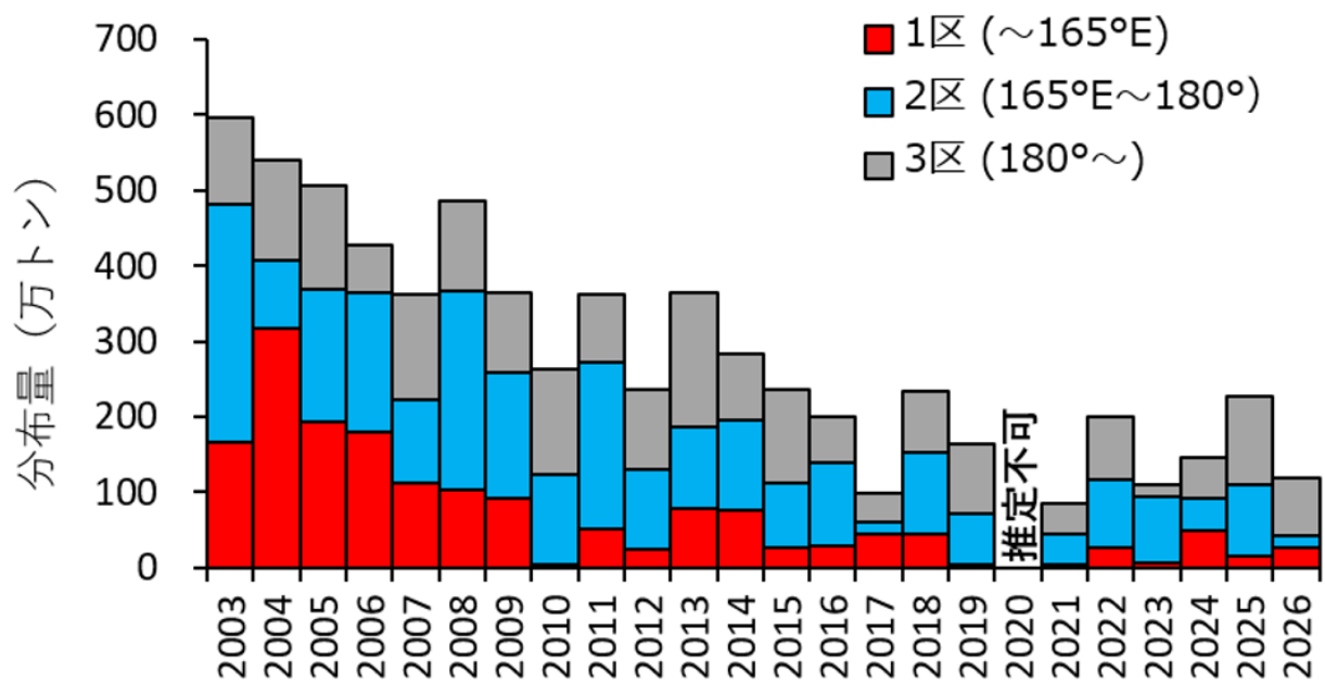
図3. サンマ資源量直接推定調査で推定された2003年～2026年の海区別サンマ分布量。2020年は調査範囲が極端に狭かったため、比較可能な指標が推定できなかった。
