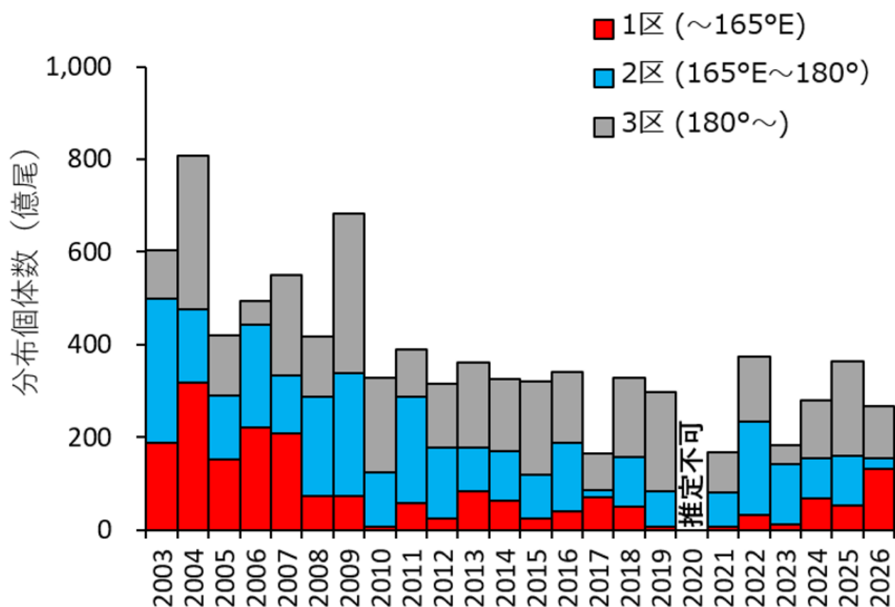
補足図 1-4. サンマ資源量直接推定調査で推定された 2003 年～2026 年の海区別のサンマ分布量。上は重量ベース、下は個体数ベースによるサンマ推定分布量。
