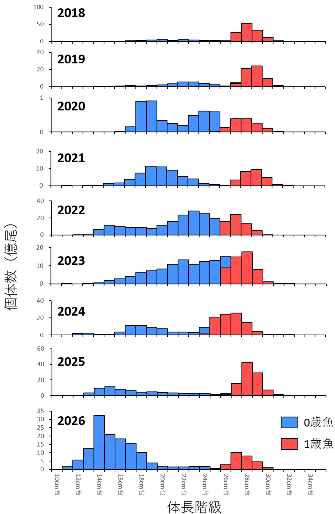
図4. サンマ資源量直接推定調査結果をもとに推定された1区と2区（180度以西）に分布していたサンマの体長組成の経年変化。
