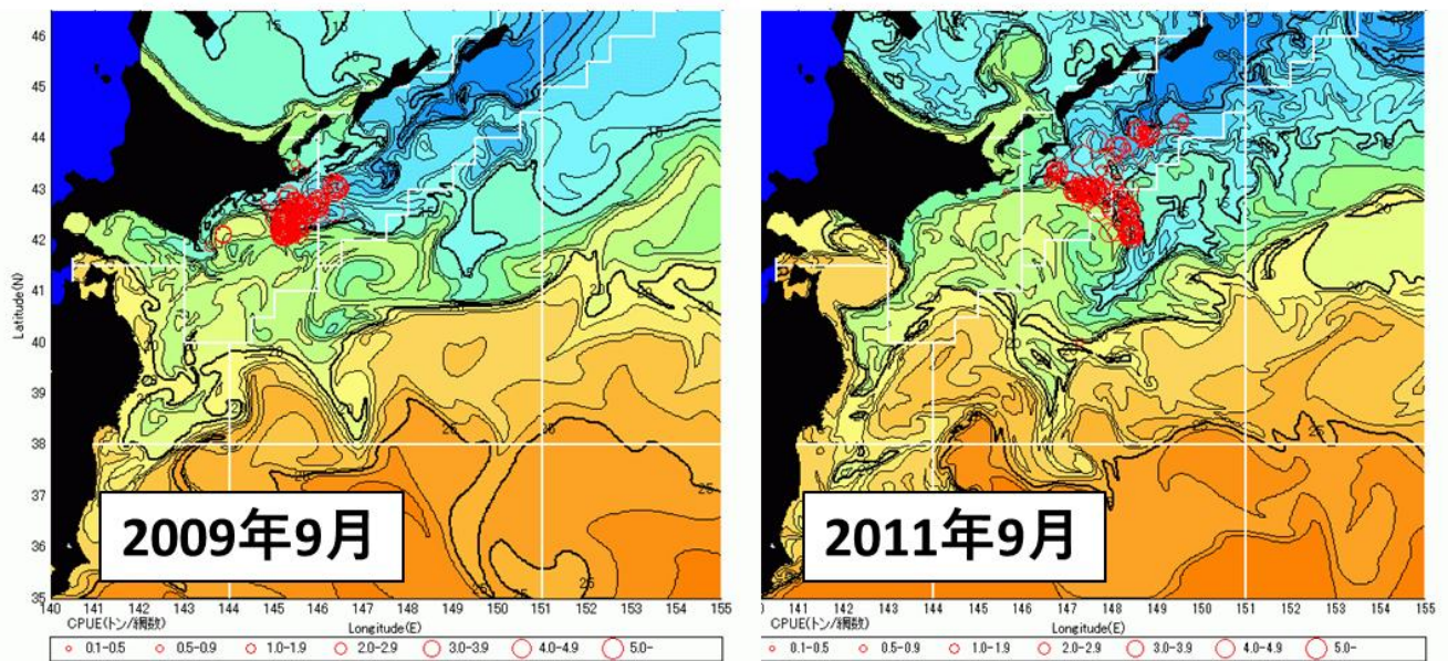
図9. 海洋環境とサンマの漁場の関係。親潮に沿って南下してきたサンマは暖水塊の縁に沿って本州東方沖に達する。その後道東沿岸に伸びた親潮に沿って魚群が道東沿岸に達するが（2009年の例）、暖水塊が道東沿岸に接すると親潮が沿岸に貫入せず、沖合に発達した親潮に沿って南下する。
