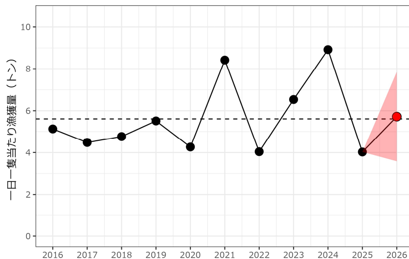
図 1. 過去 10 年間の 6～11 月の近海竿釣り船による CPUE の経年変化と予測された 2026 年の CPUE（赤マーカー）。図中の点線は過去 10 年間の平均値（2016～2025 年）、赤領域は 80%予測区間を示す。
