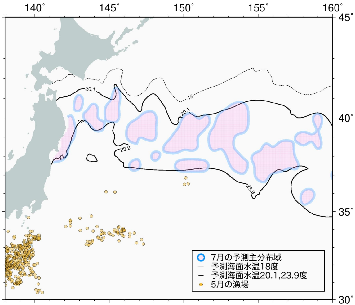
図2. 2026年7月のカツオ主分布域の予測
