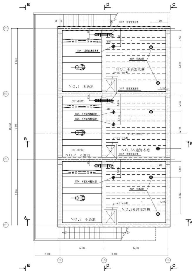
1FL+12000レベル見下ろし図
