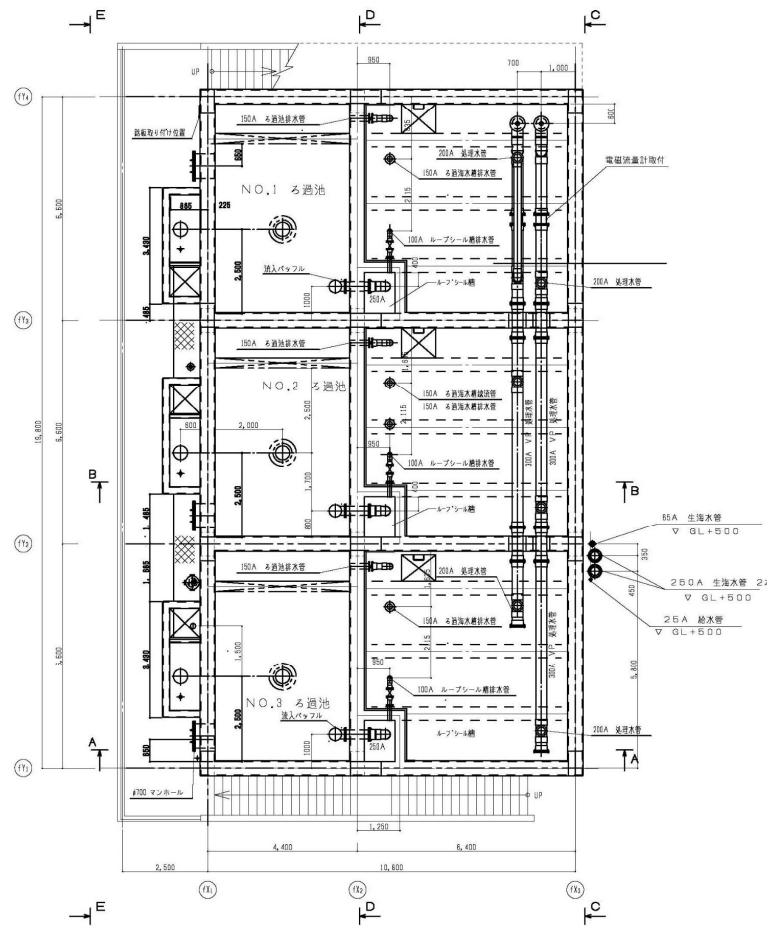
1FL+8500レベル見下ろし図
