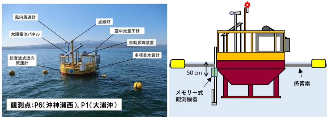
図3. 観測点 P6 に設置している大型自動観測ブイ（左）と冬季観測（10月～3月）における観測機器の設置概要（右）
